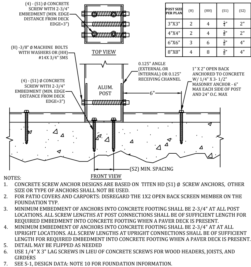
G1 ALUM. POST CONNECTION DETAIL SCALE: N.T.S.
