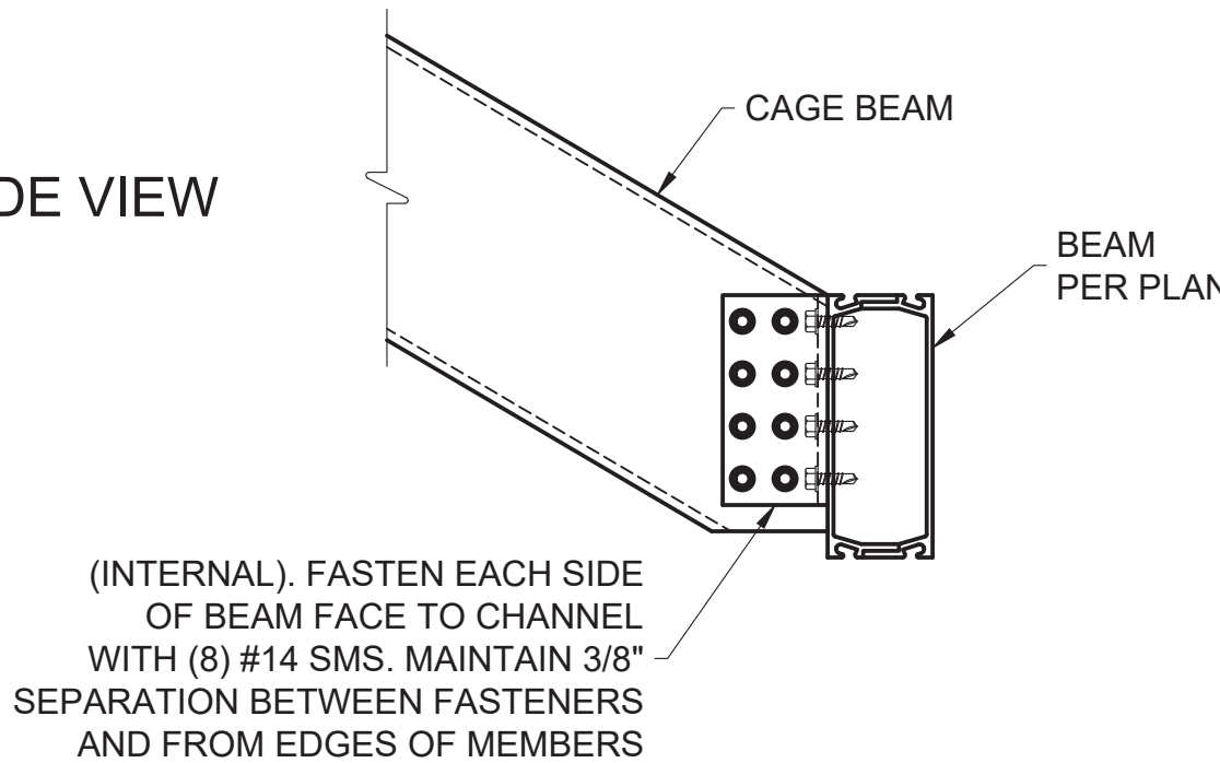
BEAM TO EDGE BEAM DETAIL SCALE: N.T.S.
