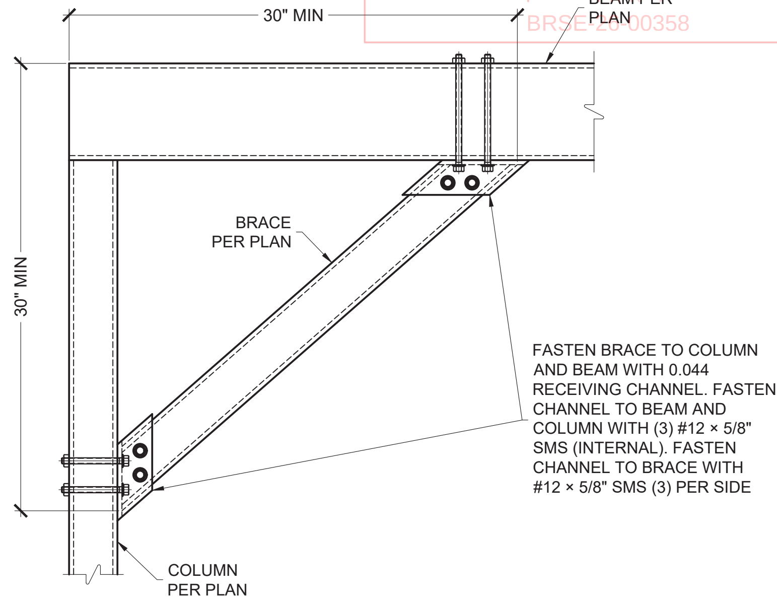
K-BRACE DETAIL SCALE: N.T.S.
