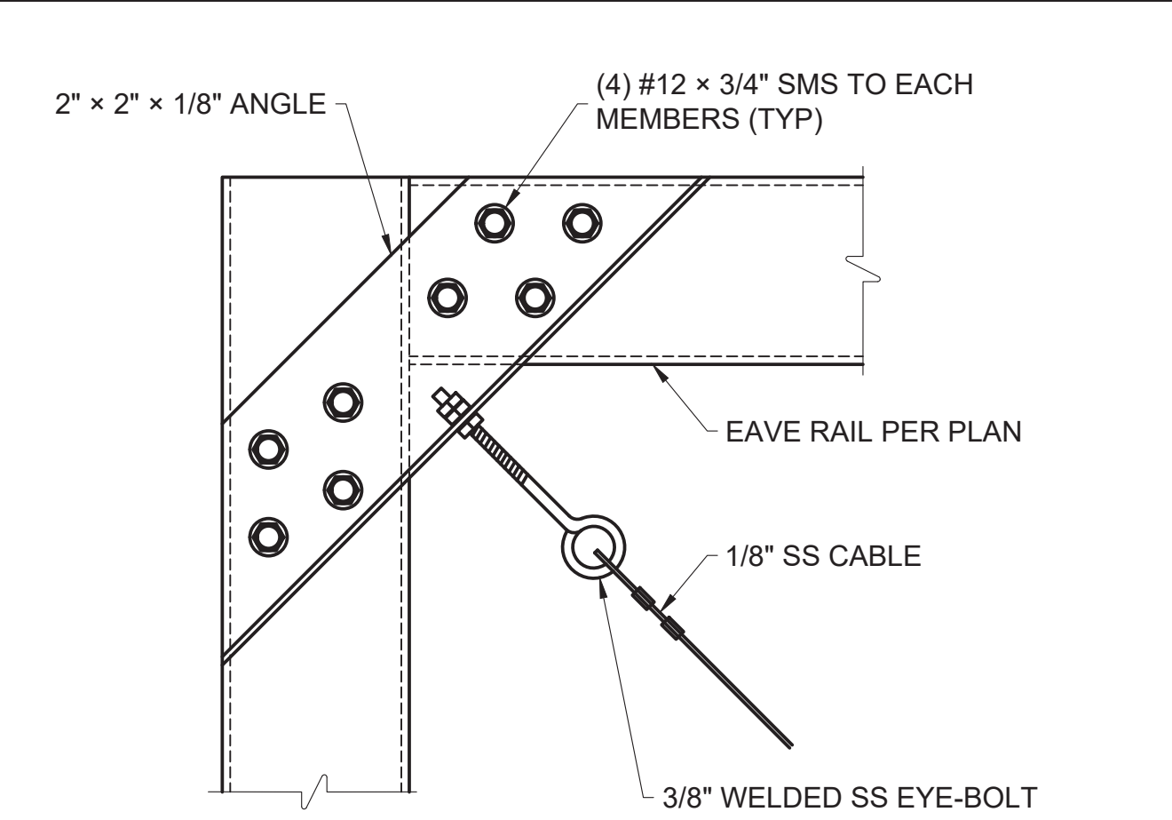
CABLE TO FRAME CONNECTION SCALE: N.T.S.
