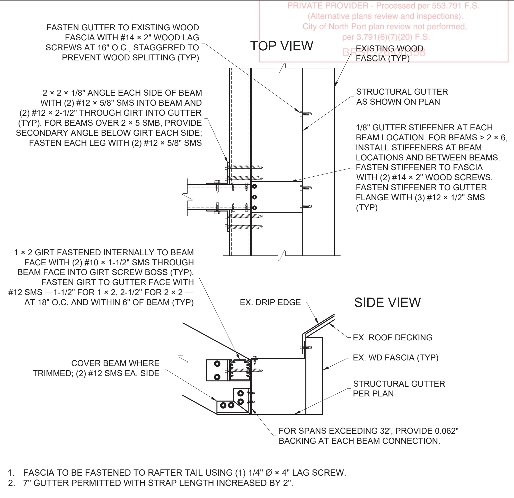
BEAM TO GUTTER CONNECTION SCALE: N.T.S.
