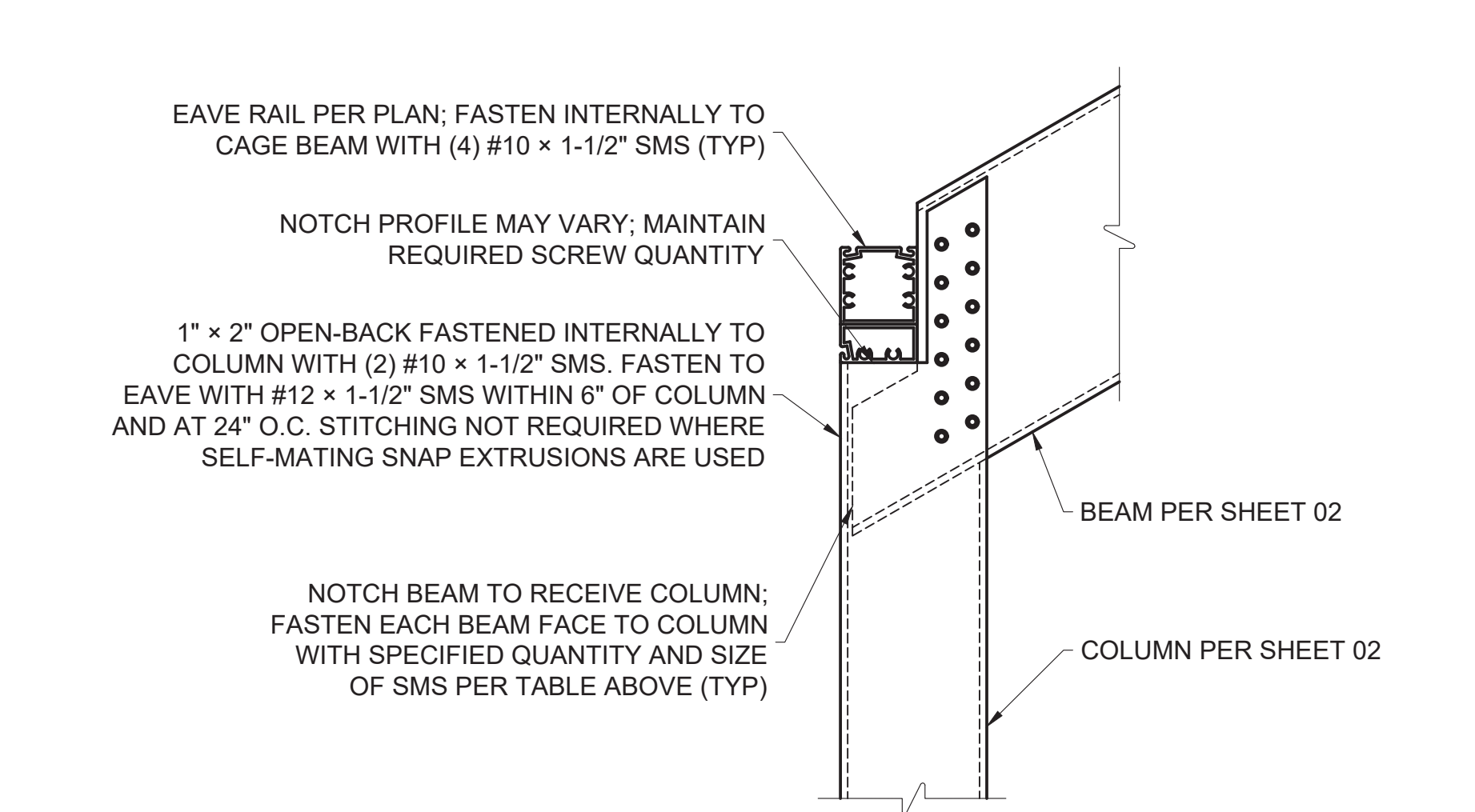
COLUMN TO BEAM CONNECTION SCALE: N.T.S.
