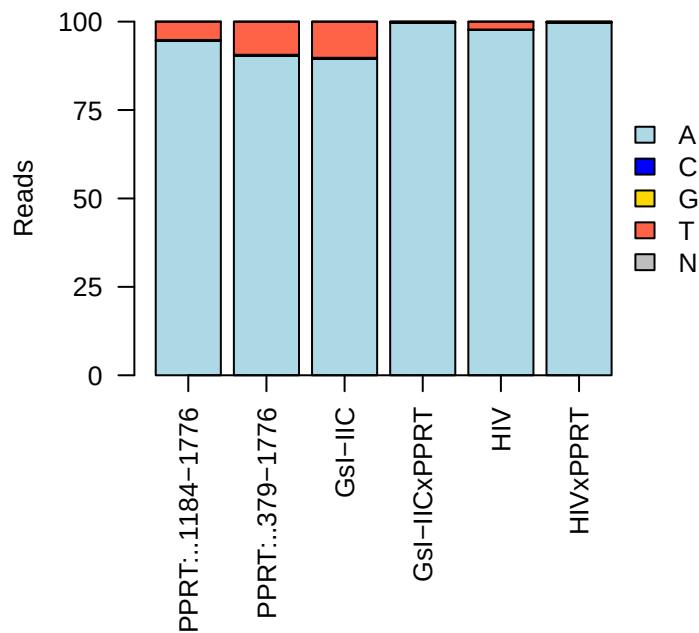
Pos31 (A→T)
