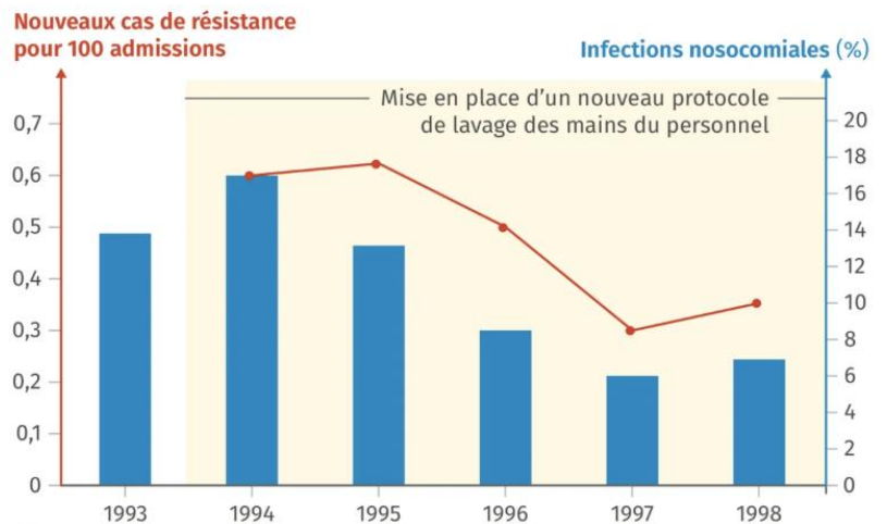
Document 1: Résistance de S. aureus à un antibiotique en milieu hospitalier. Infection nosocomiales = infection apparue au cours ou à la suite d'une hospitalisation
