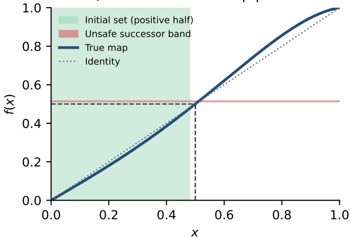
Quadratic invariant: |x| \leq 1/2
