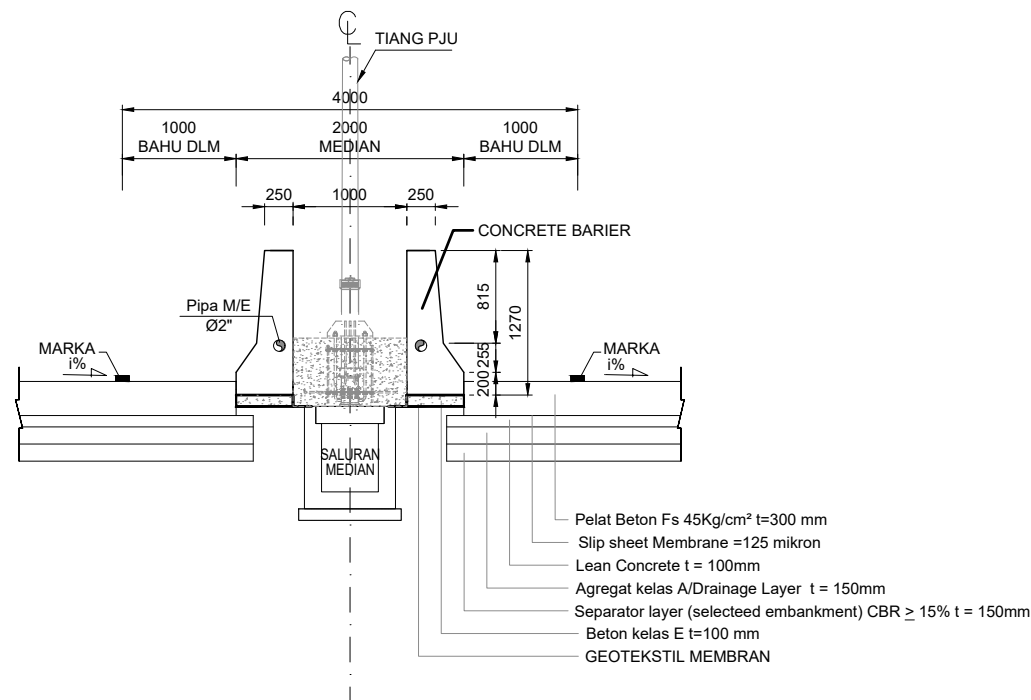
DETAIL MEDIAN PADA SUPERELEVASI DENGAN TIANG PU
