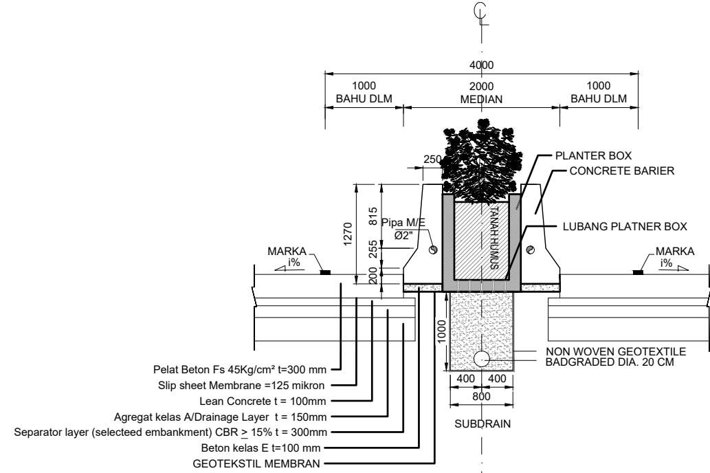
DETAIL MEDIAN PADA GALIAN DENGAN TANAMAN
