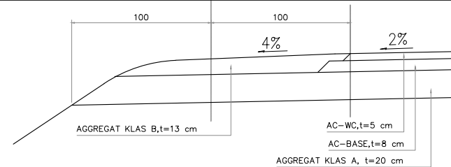
DETAIL-B SKALA 1:40
