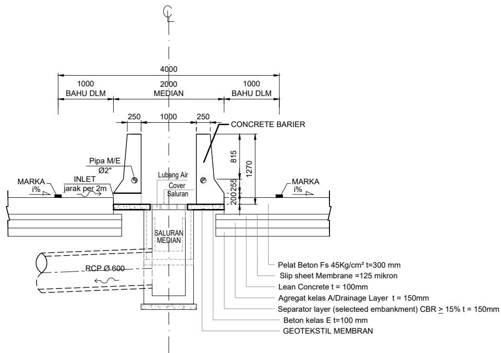
DETAIL MEDIAN PADA SUPERELEVASI
