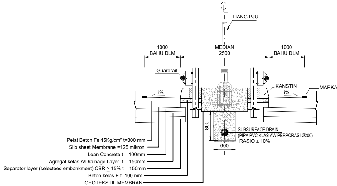
DETAIL C MEDIAN AKSES DENGAN TIANG PJU
