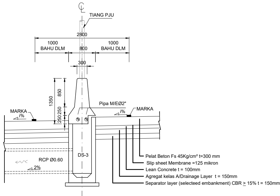
DETAIL E MEDIAN AKSES KONDISI SUPERELEVASI
