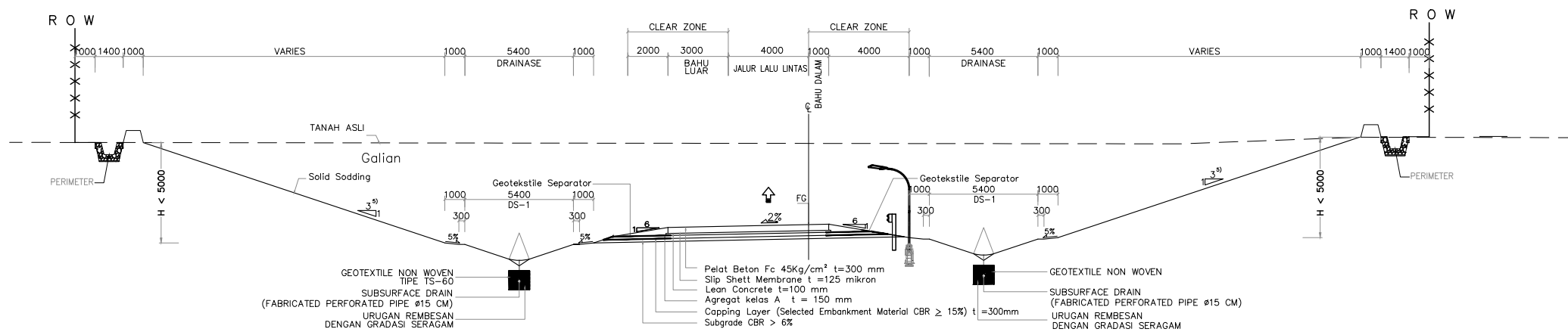
TIPIKAL POTONGAN MELINTANG RAMP INTERCHANGE PASIR BARAT PADA DAERAH GALIAN RAMP-2 PASIR BARAT STA.0+325 - STA.0+500
