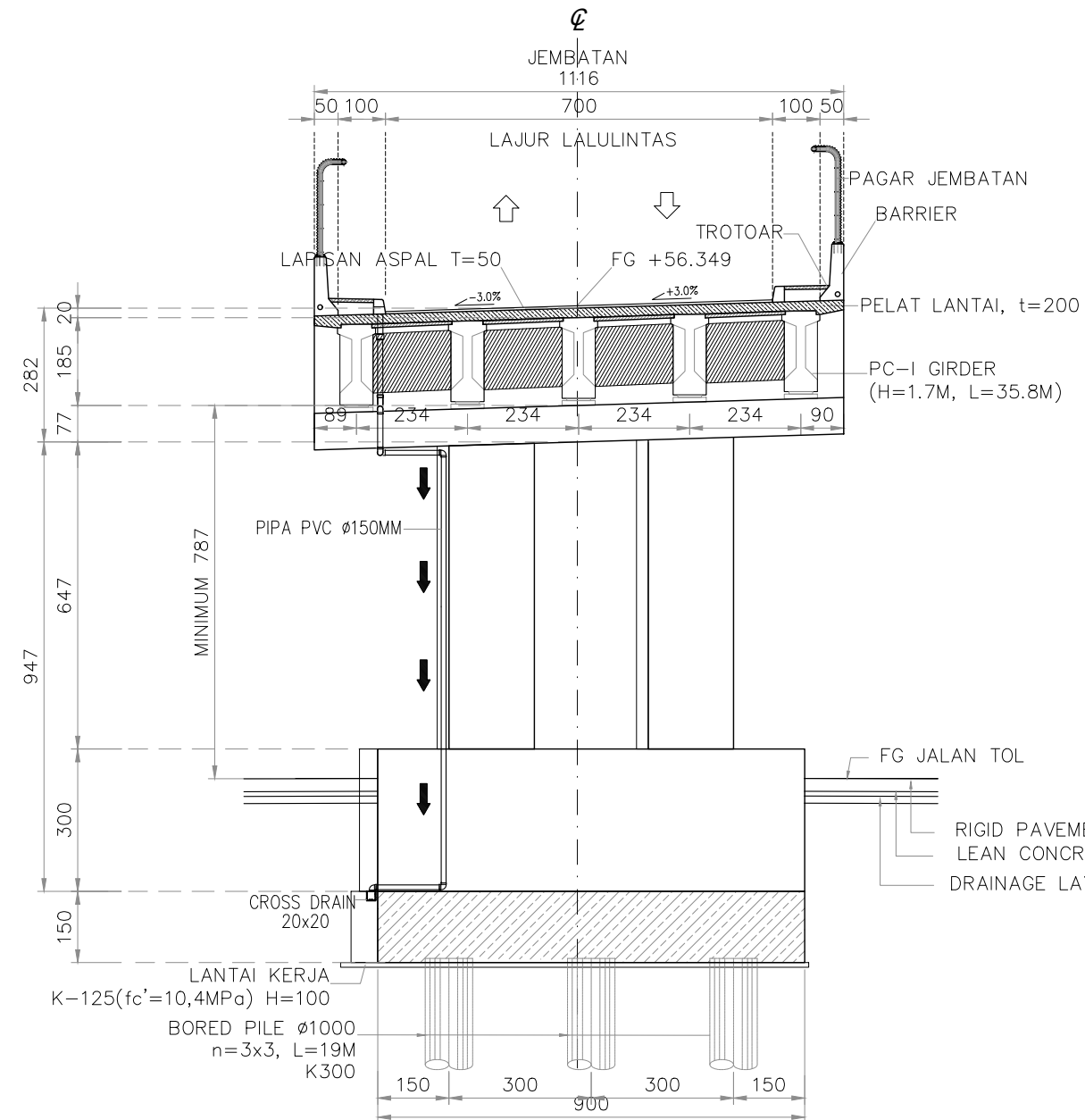
TIPIKAL STRUKTUR JEMBATAN OVERPASS JALAN NASIONAL SKALA 1 : 150
