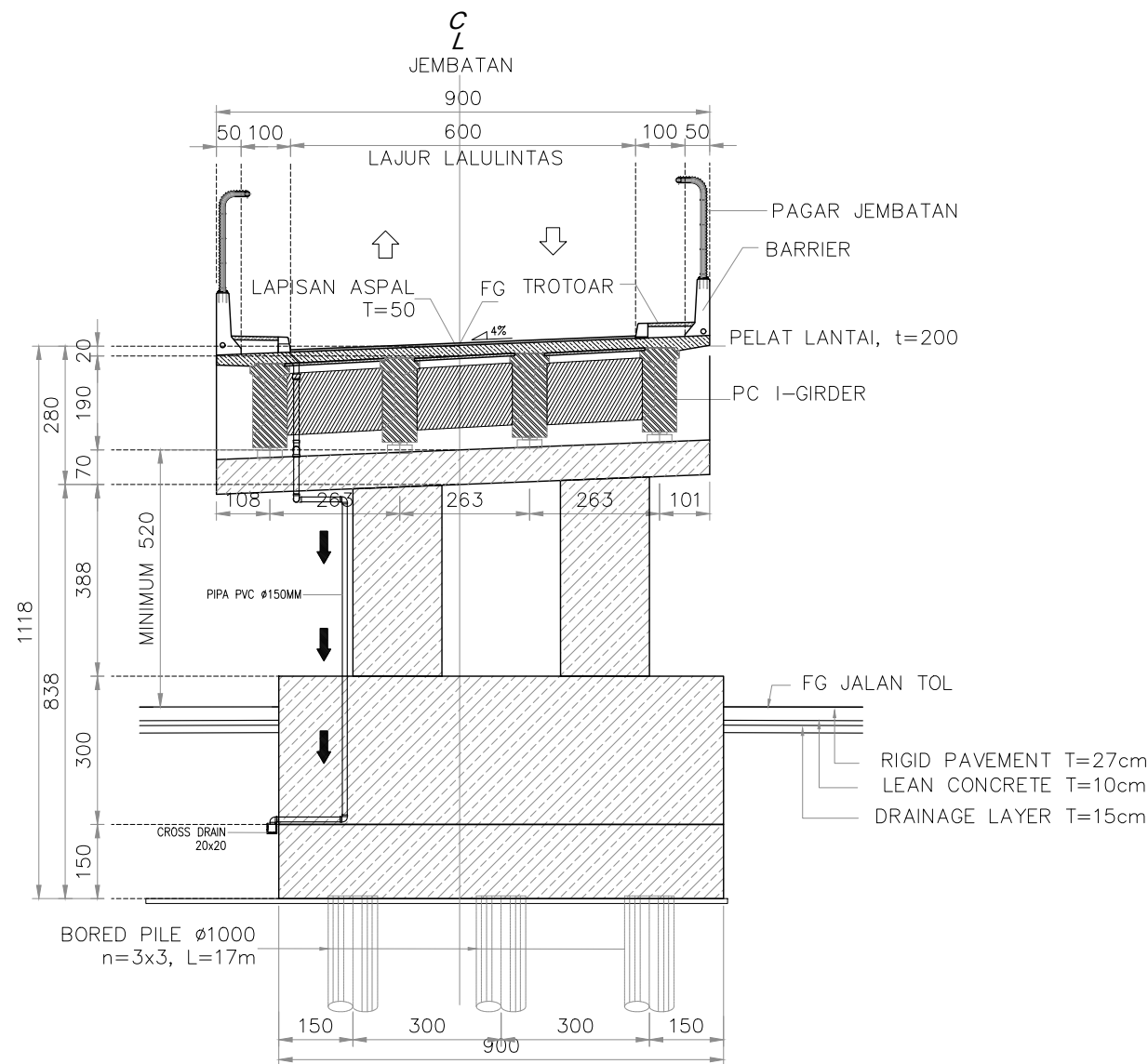
TIPIKAL STRUKTUR JEMBATAN OVERPASS JALAN KABUPATEN SKALA 1 : 150
