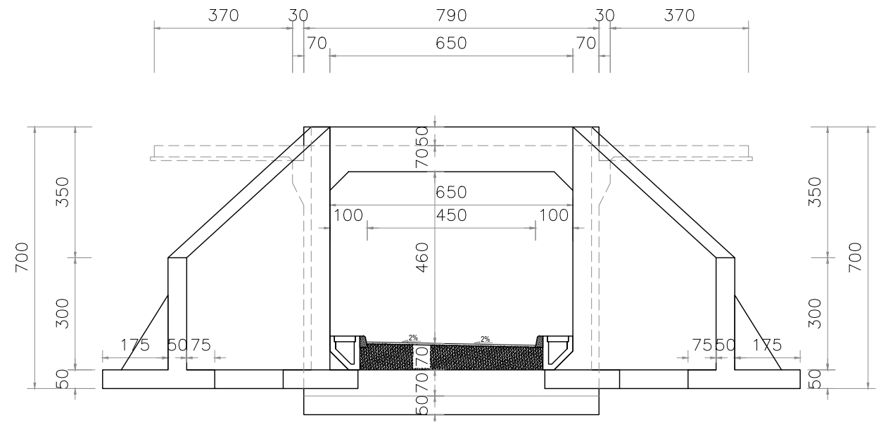
POTONGAN MELINTANG UNDERPASS TYPE JALAN DESA
