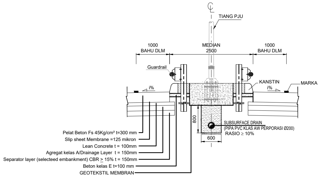
DETAIL MEDIAN AKSES DENGAN TIANG PLU
