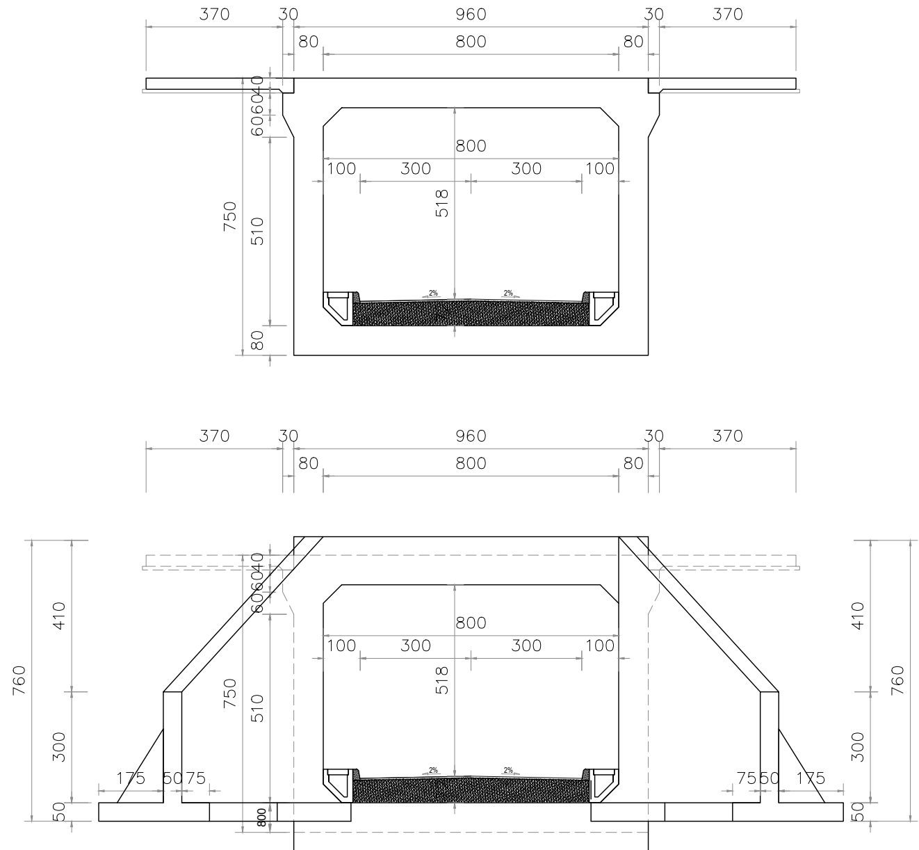
POTONGAN MELINTANG UNDERPASS TYPE JALAN KABUPATEN
