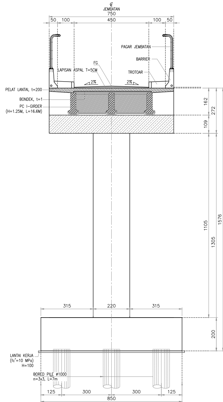
TIPIKAL STRUKTUR JEMBATAN OVERPASS JALAN DESA SKALA 1 : 150
