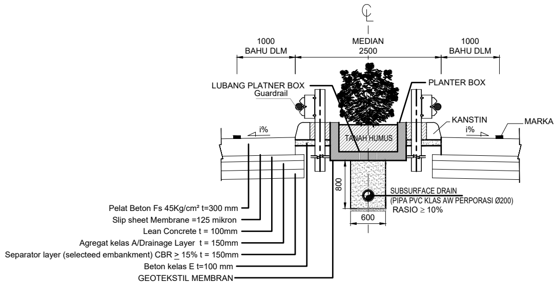
DETAIL C MEDIAN AKSES DENGAN TANAMAN
