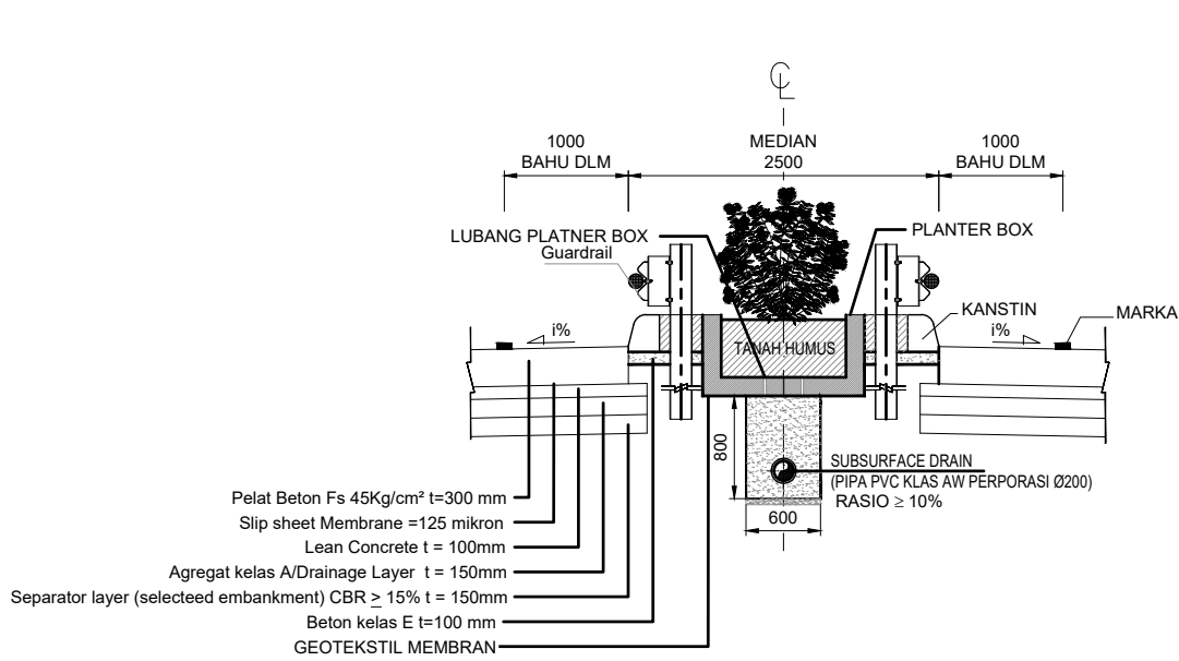
DETAIL MEDIAN AKSES DENGAN TANAMAN
