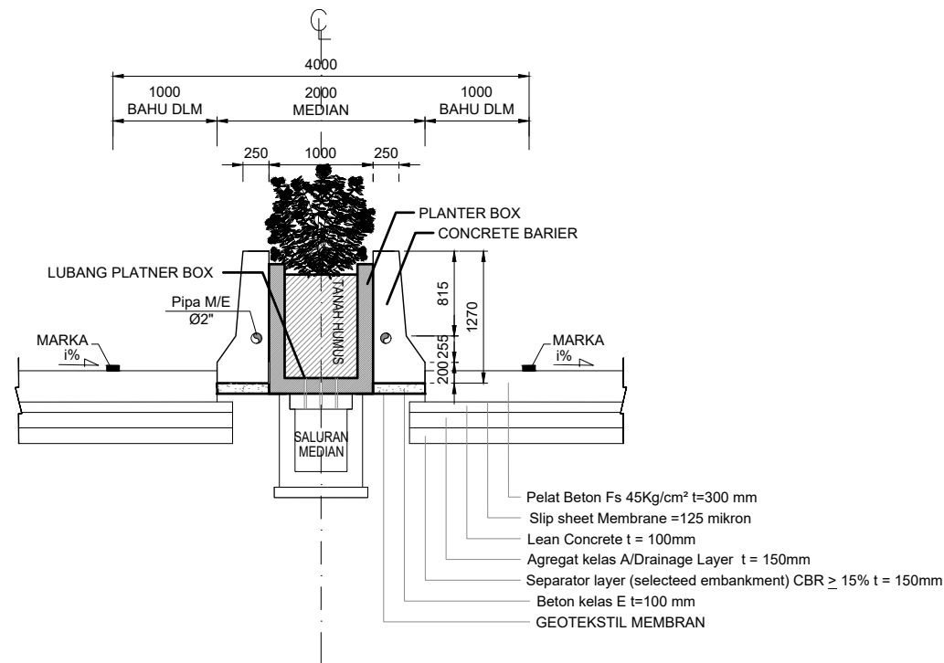
DETAIL MEDIAN PADA SUPERELEVASI DENGAN TANAMAN
