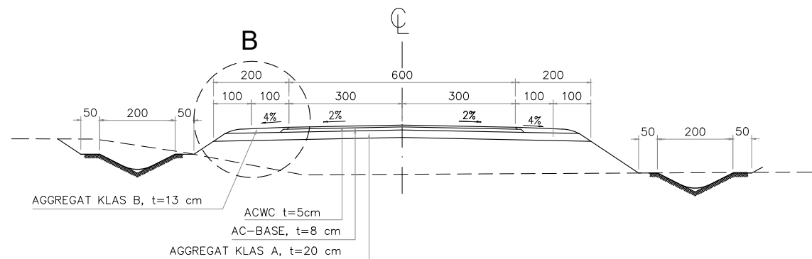
JALAN KABUPATEN TIPE-1 SKALA 1:150
