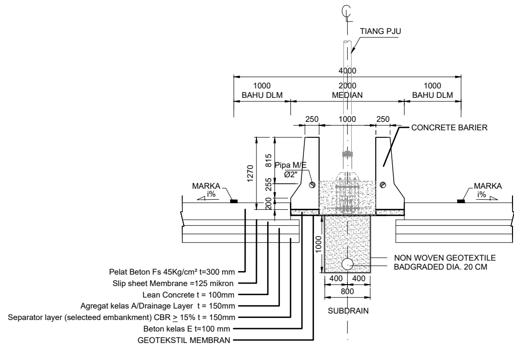
DETAIL MEDIAN PADA TIMBUNAN DENGAN TIANG PJU
