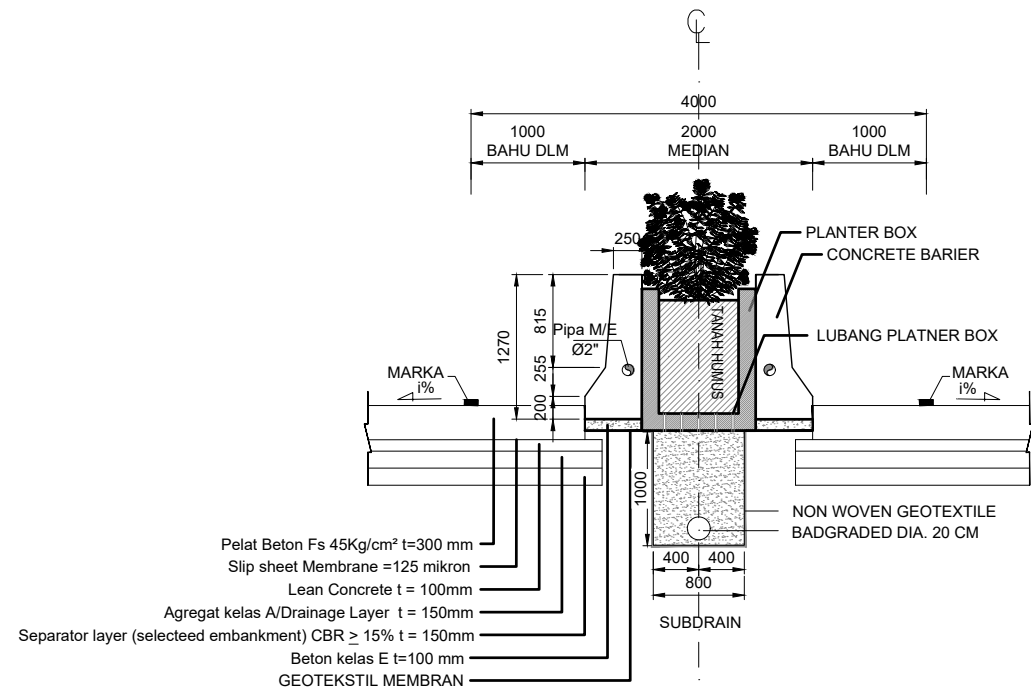
DETAIL MEDIAN PADA TIMBUNAN DENGAN TANAMAN
