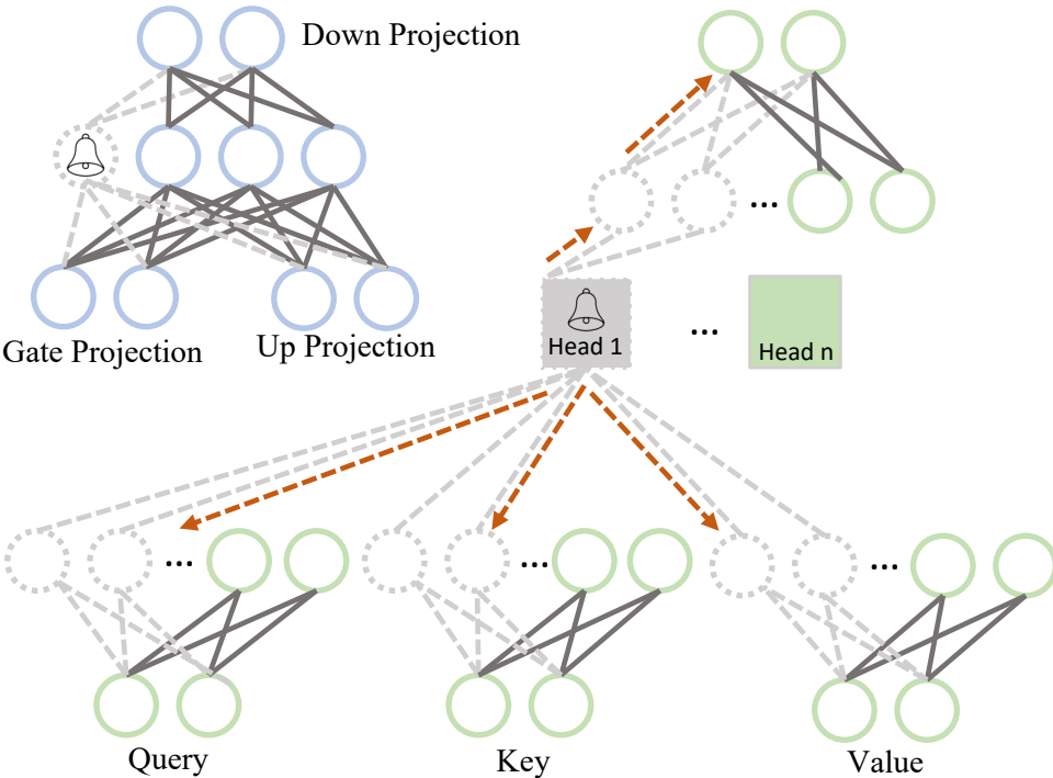
Group Type A: MLP
