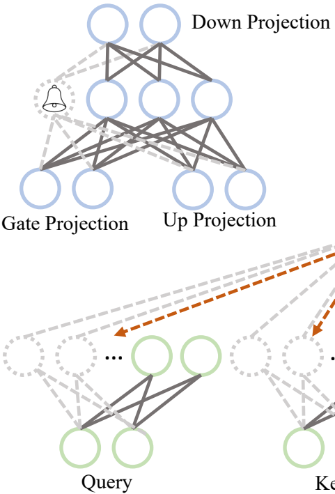
Group Type A: MLP
