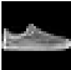
Sandal (Sneaker)
