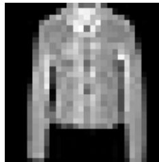
Pullover (Pullover)
