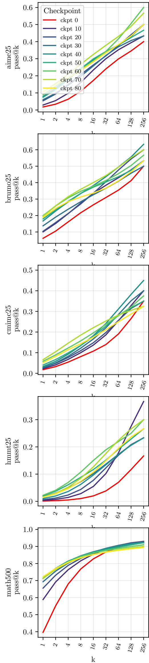
Qwen2.5-7B, GSPO
