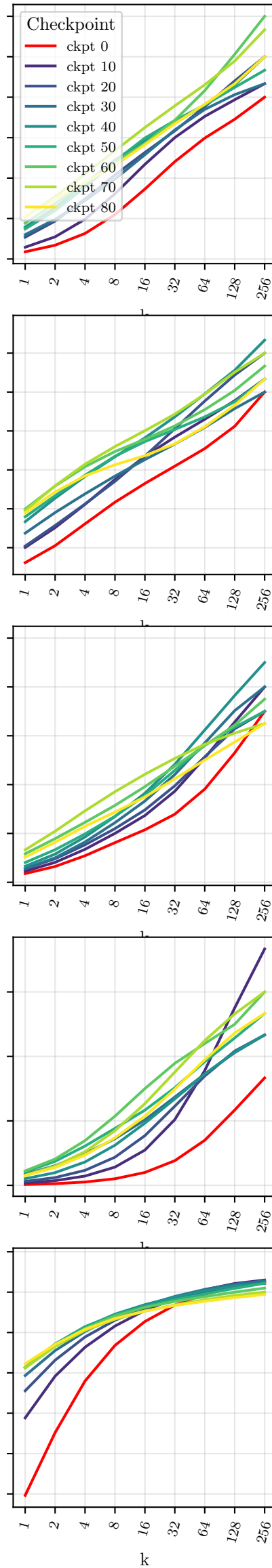
Qwen2.5-7B, GSPO
