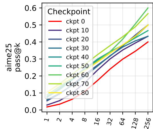
Qwen2.5-7B, GSPO
