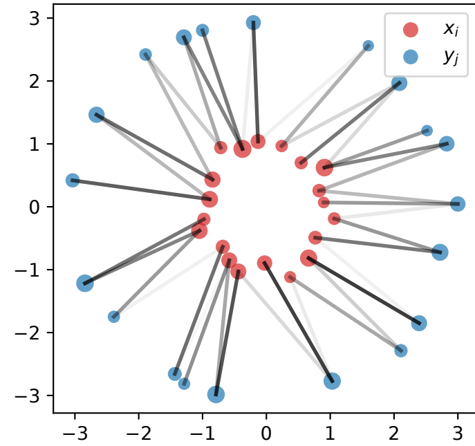
Problème et plan optimal P
