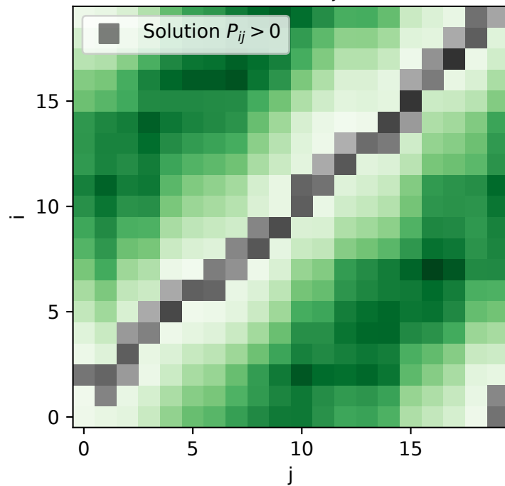
Matrice de coût c(x_i, y_j) et solution P
