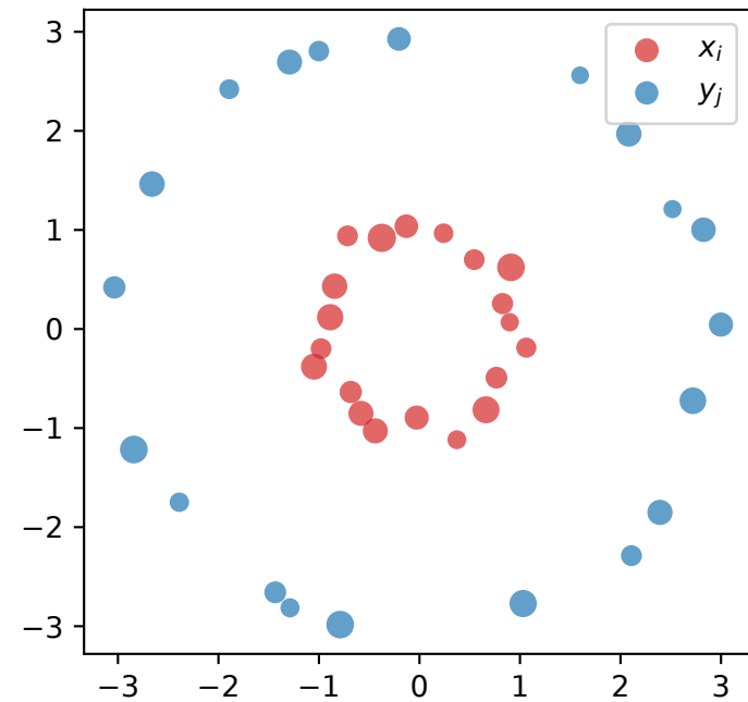
Problème de Kantorovitch
