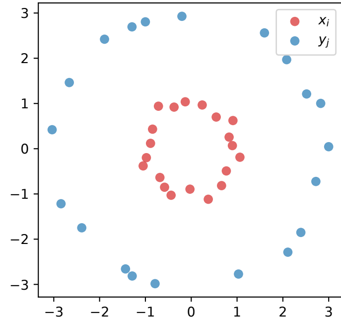
Problème de Monge
