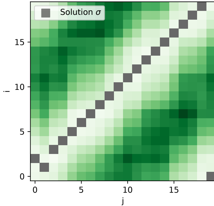
Matrice de coût c(x_i, y_j) et solution \sigma
