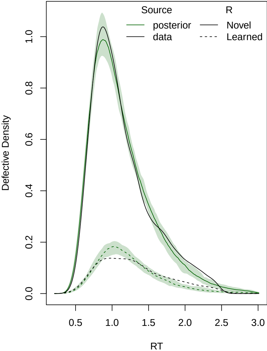
S=Novel
