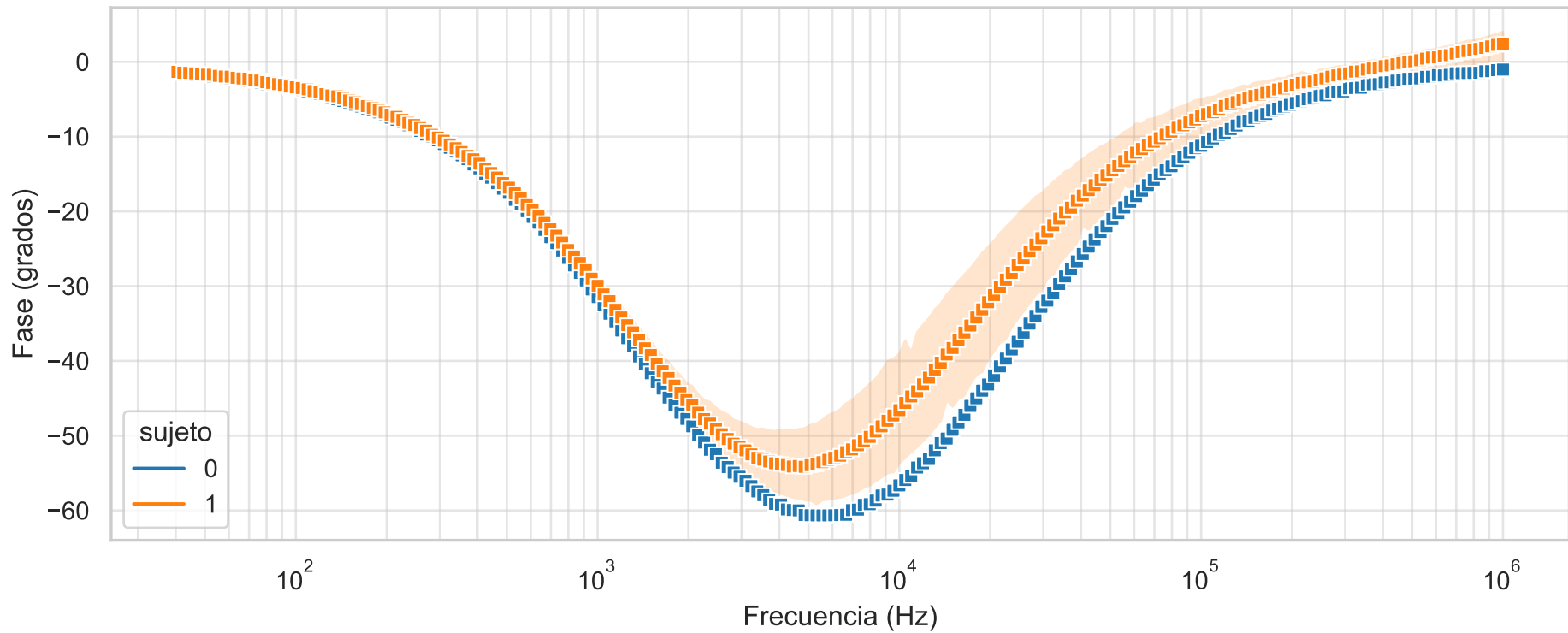
Respuesta en Frecuencia: Fase
