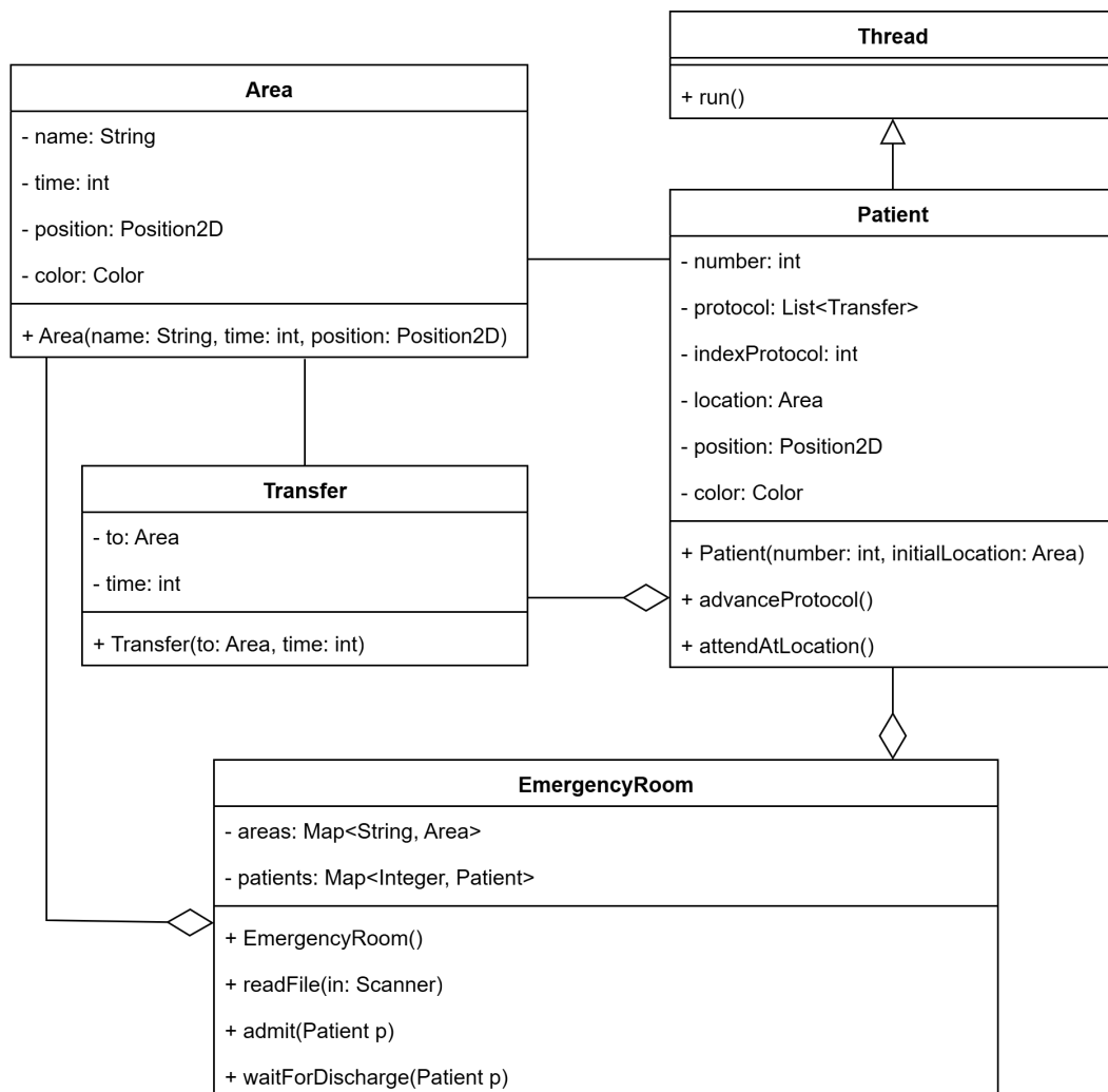
Figura 2: Diagrama de clases del simulador del servicio de Urgencias.
