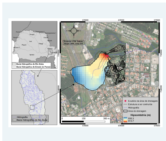
Mapa hipsométrico das áreas de drenagem relevantes para o estudo. Figura 6 do relatório, p. 13.
