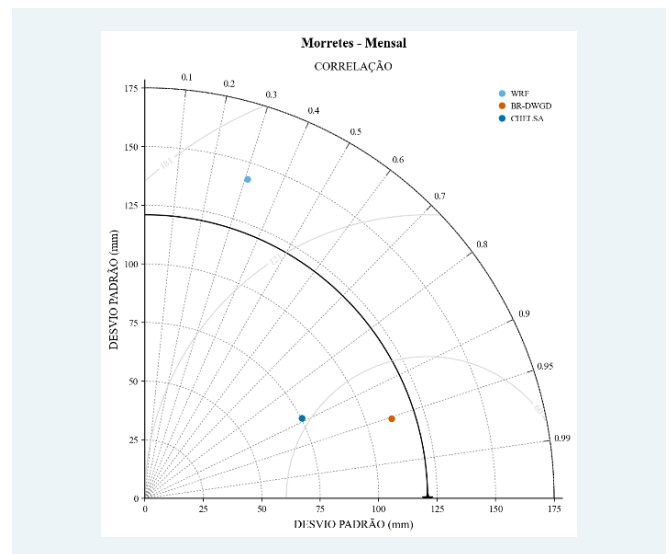
Diagrama de Taylor para Morretes, escala mensal. Detalhe da figura 6 do manuscrito, p. 7.
