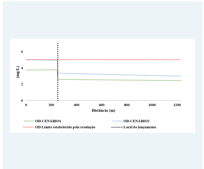
Concentração simulada de oxigênio dissolvido ao longo do canal. Figura 7-4 do relatório, p. 31.
