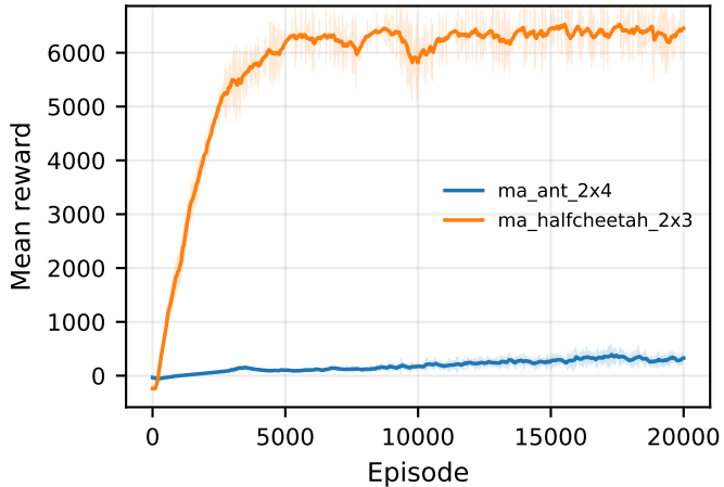
MAAC
