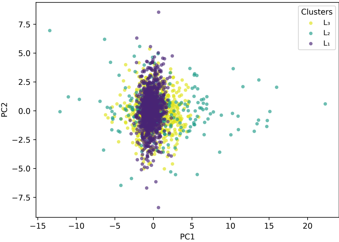
GMM (subset) PC1 vs PC2 | k=3
