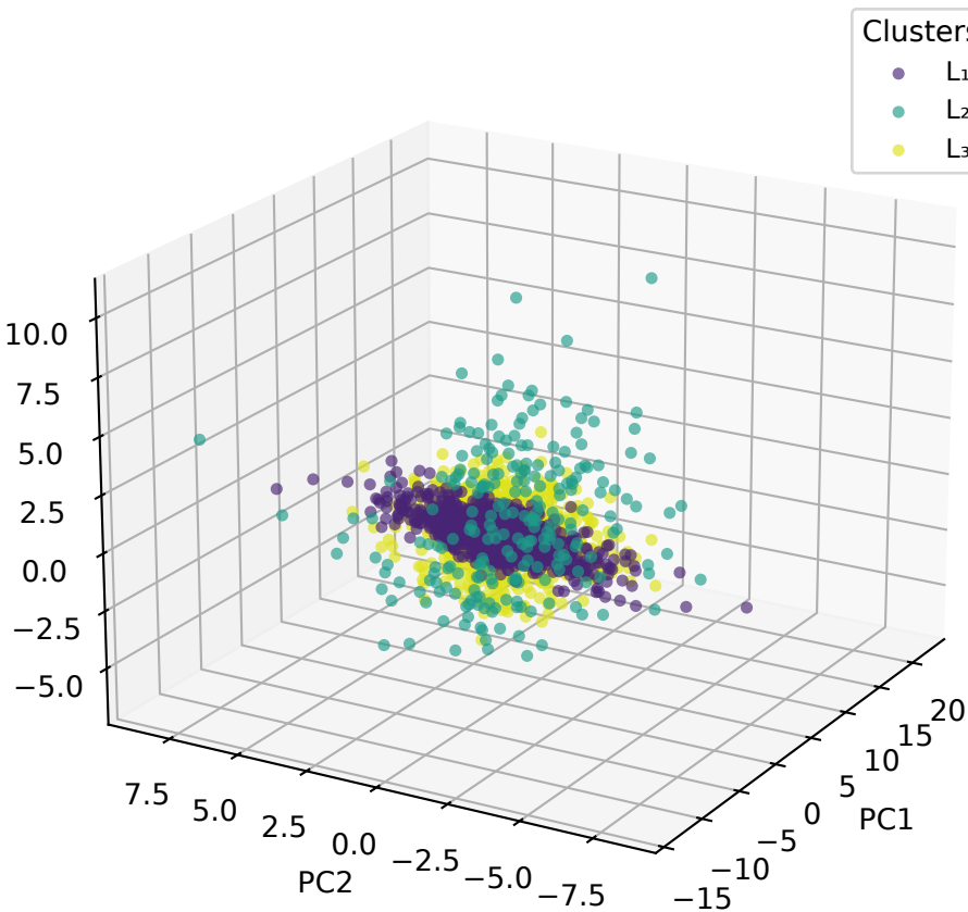
GMM (subset) k=3 | elev=20 azim=210
