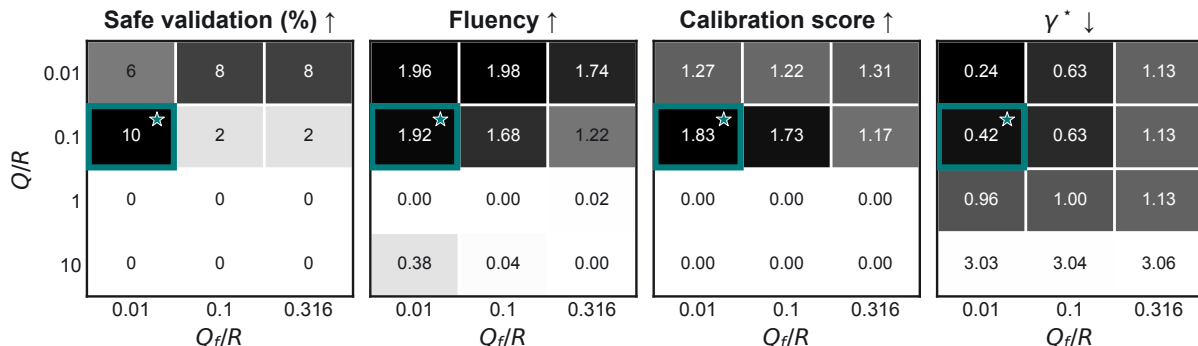
Llama-3.2-3B
