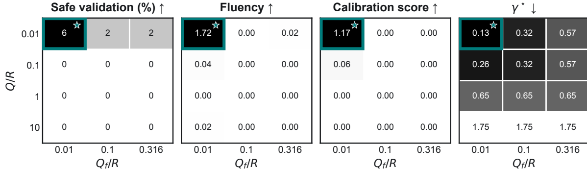
Llama-3.2-1B
