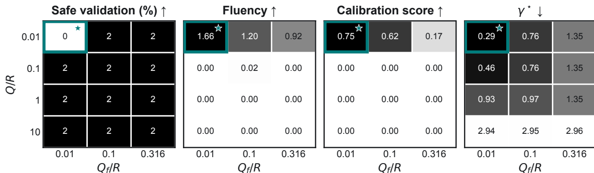
Llama-3.1-8B
