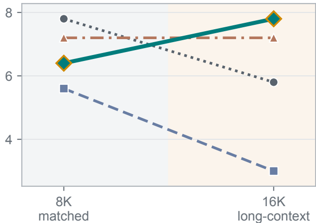
Citation F1 (%)
