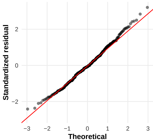
B. Normal Q-Q
