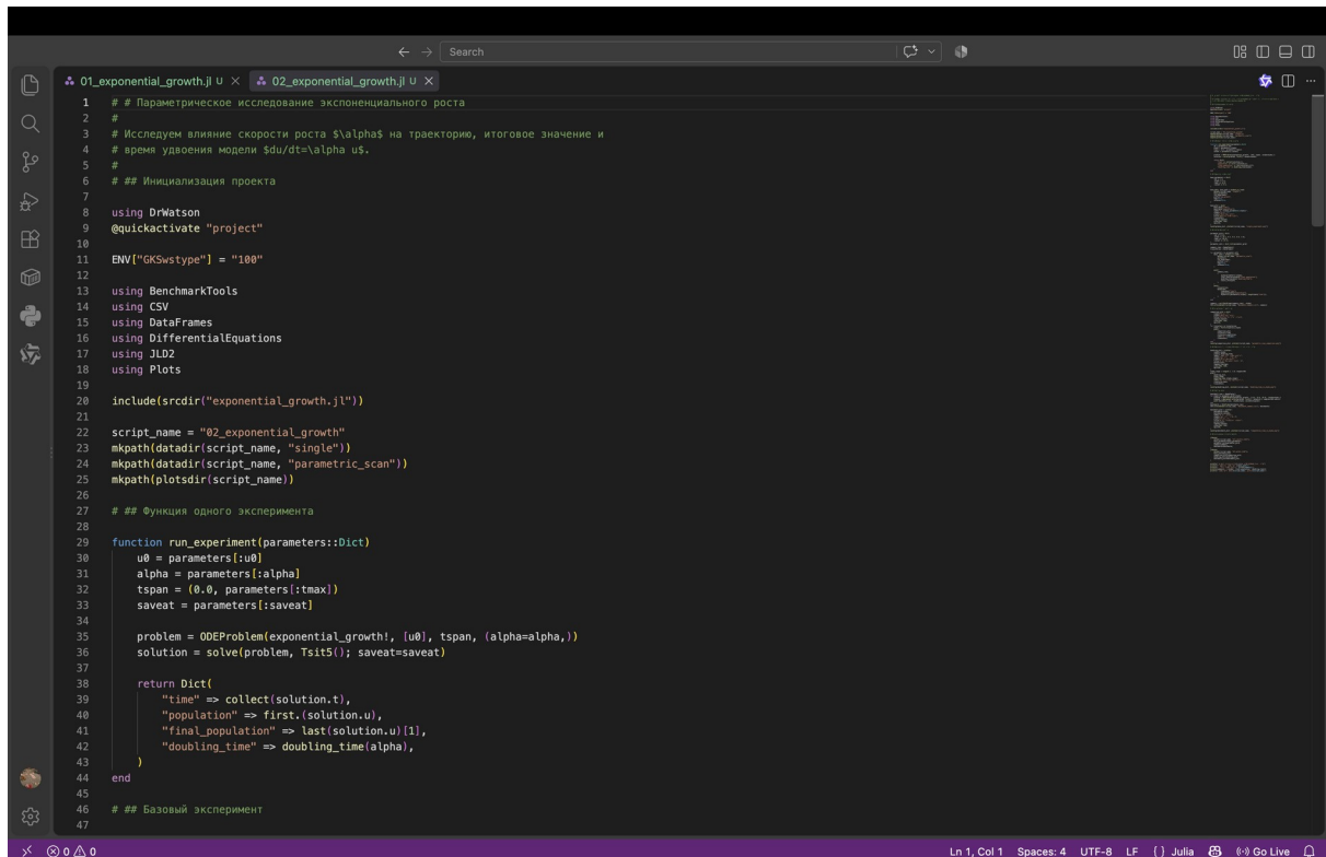
Рисунок 5: Фрагмент сценария серии экспериментов
