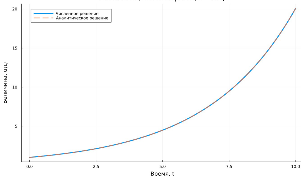
Рисунок 4: Численное и аналитическое решения при \alpha = 0,3
