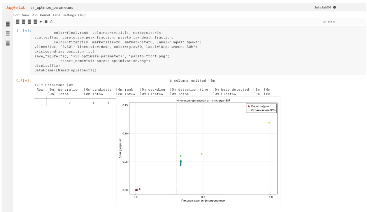
Рисунок 16: Notebook оптимизации
