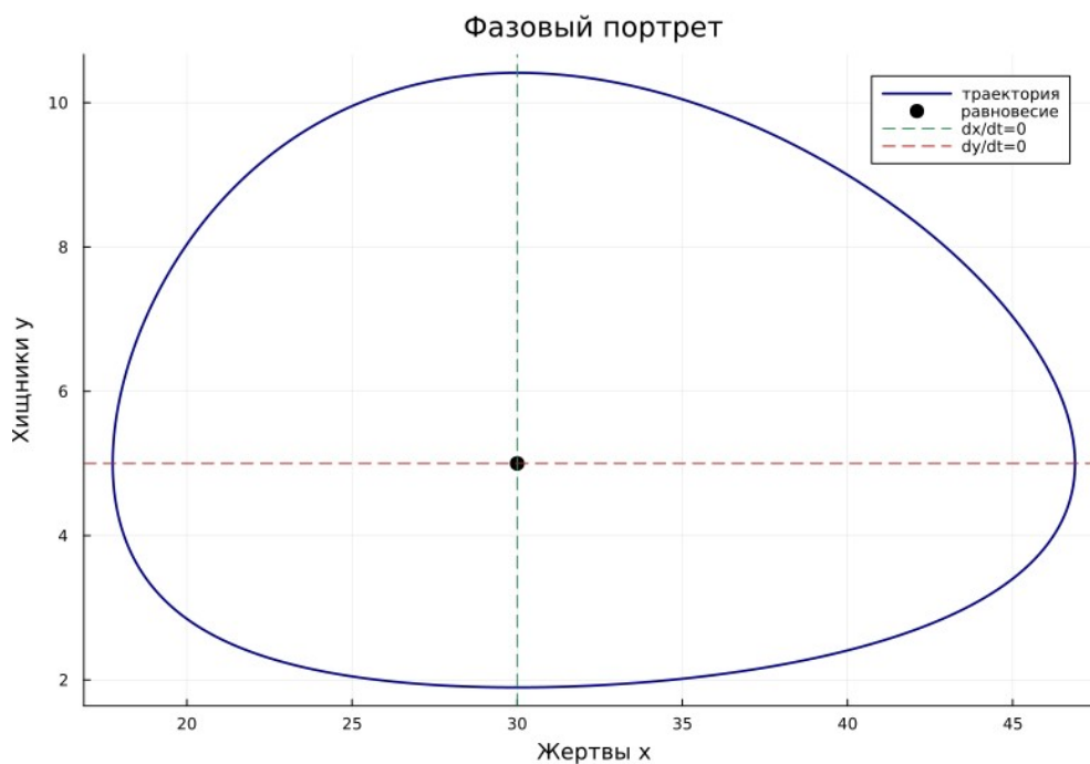
Рисунок 11: Замкнутая орбита вокруг равновесия
