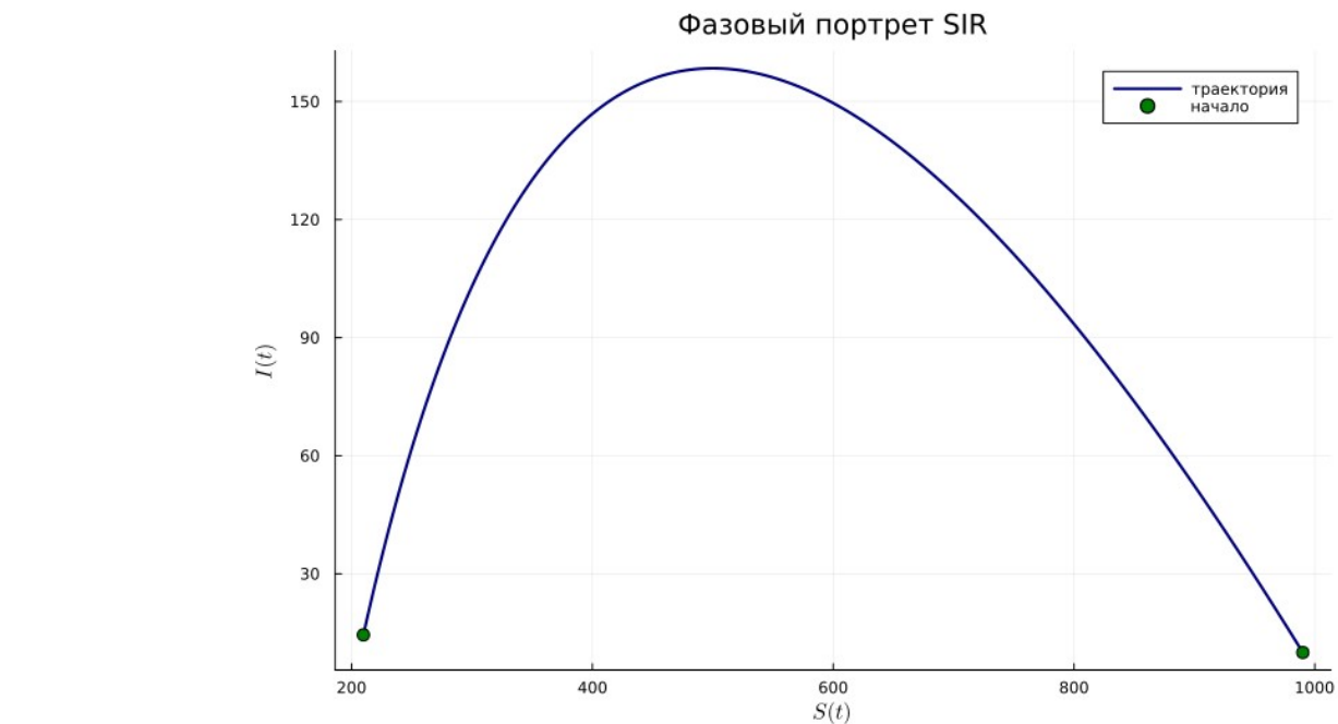
Рисунок 6: Фазовая траектория SIR
