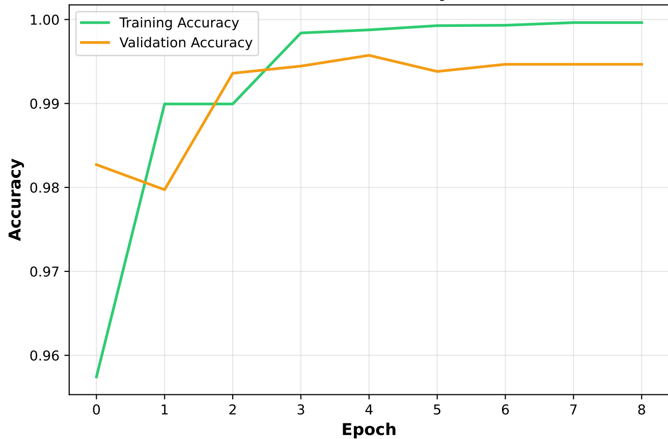
GRU - Accuracy
