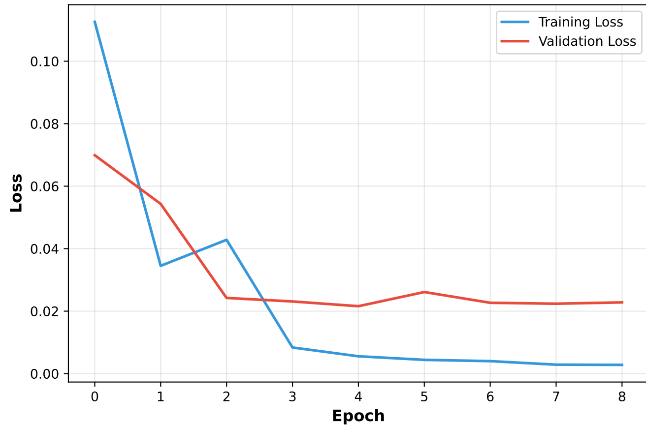
GRU - Loss
