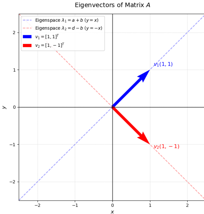
Fig. 1.2.10.1 Eigen vectors plotted
