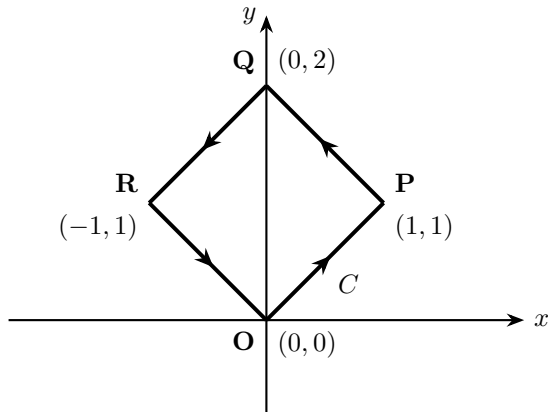
Fig. 1.2.5.1 Contour C
