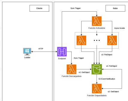
Figura: Arquitectura Solución 2
