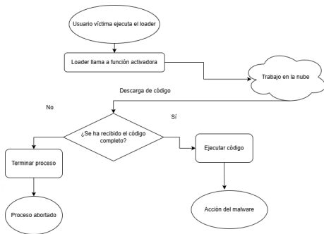
Figura: Flujo operacional en el lado del cliente
