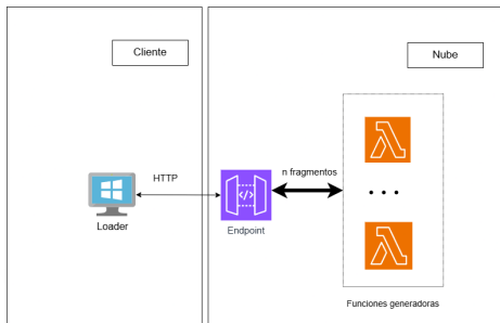
Figura: Arquitectura Solución 1
