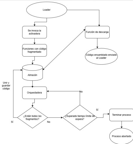
Figura: Flujo operacional en el lado del servidor
