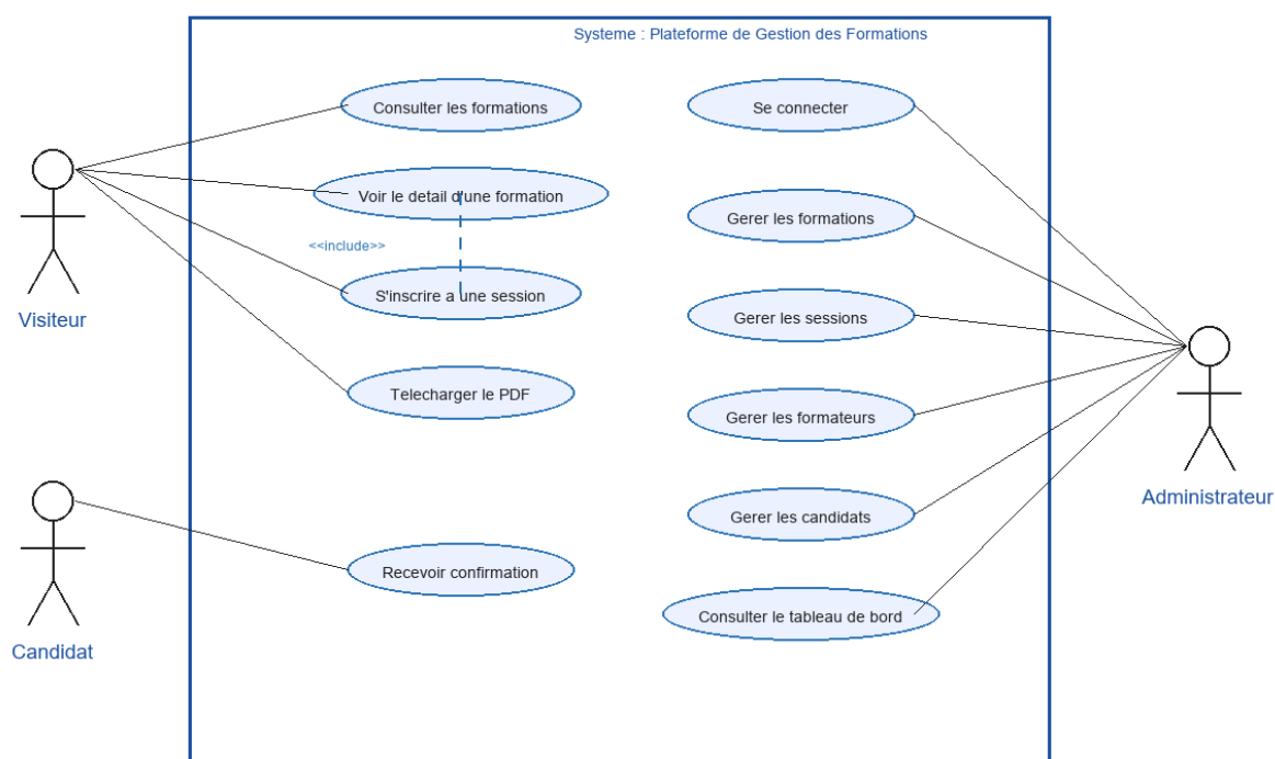
Diagramme de Cas d'Utilisation
