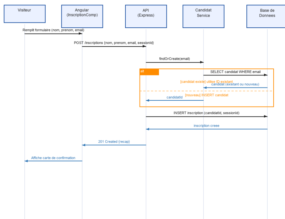
Diagramme de Sequence - Inscription a une Session
