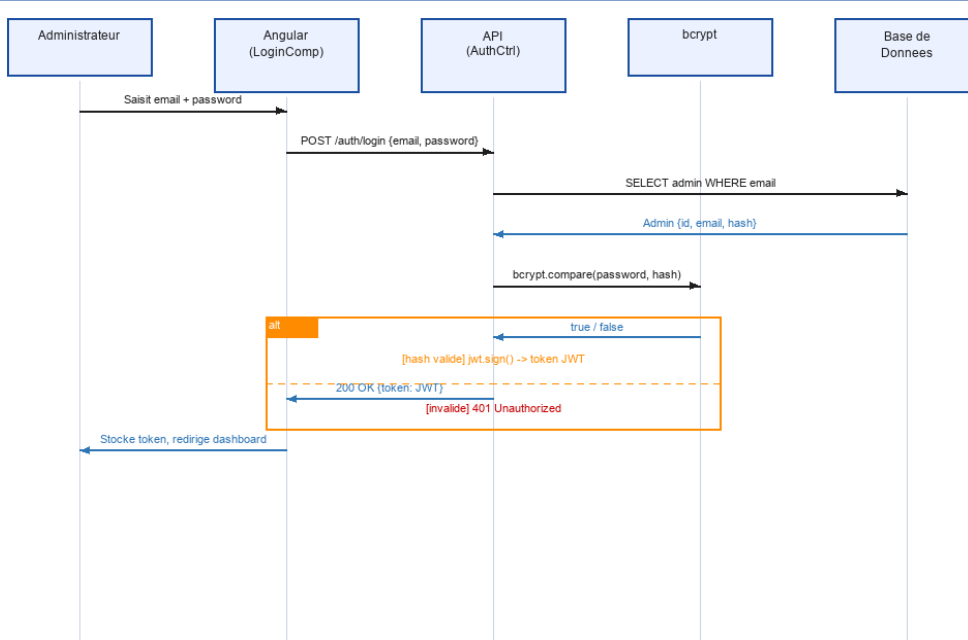
Figure 13 : Diagramme de séquence système — Login Admin
