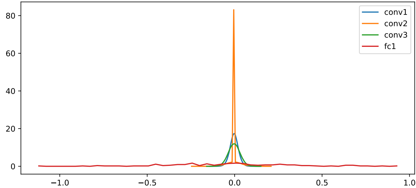
Gradient distributions - ReLU
