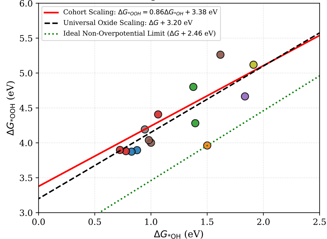
(d) Structural-Electronic Activity Correlation
