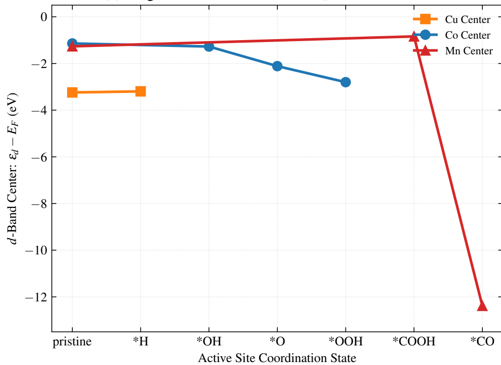
(d) Progression of d-Band Center \epsilon_d Across Adsorbates
