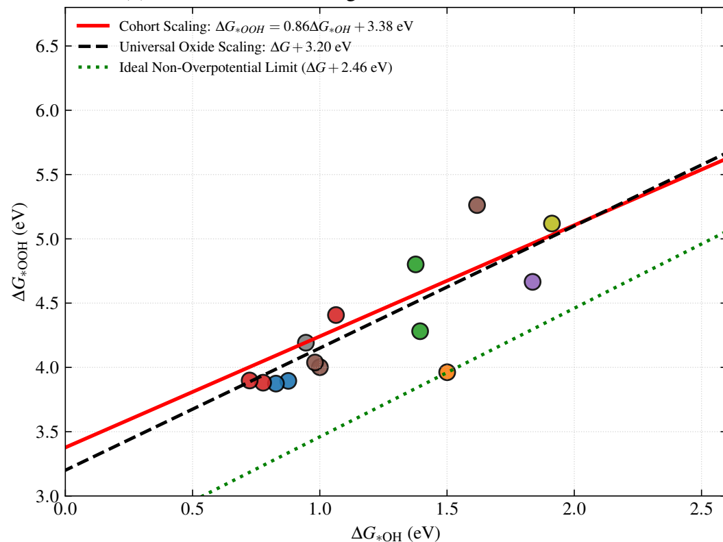
(d) Structural-Electronic Activity Correlation
