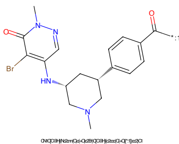
Figure 38: POI - PROTAC ID: 360
