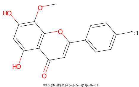
Figure 310: POI - PROTAC ID: 471
