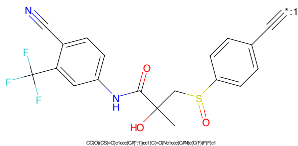
Figure 894: POI - PROTAC ID: 682
