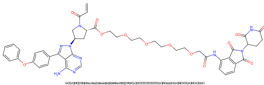
Figure 97: PROTAC - PROTAC ID: 402
