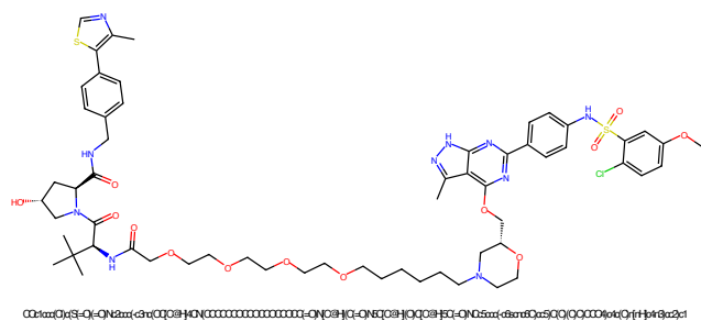
Figure 373: PROTAC - PROTAC ID: 487
