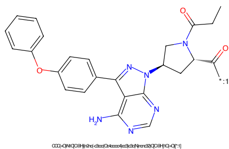
Figure 118: POI - PROTAC ID: 414
