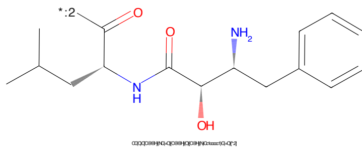
Figure 460: E3 - PROTAC ID: 509
