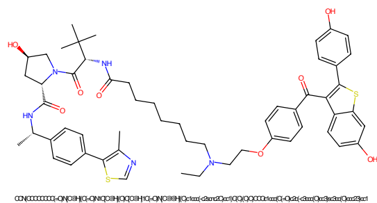
Figure 481: PROTAC - PROTAC ID: 515
