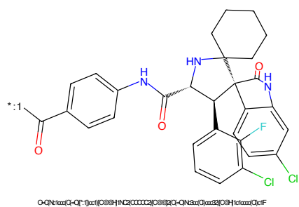
Figure 838: POI - PROTAC ID: 658
