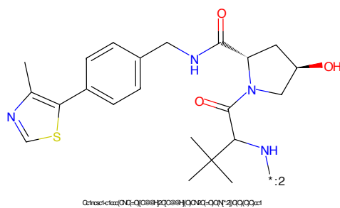
Figure 200: E3 - PROTAC ID: 435
