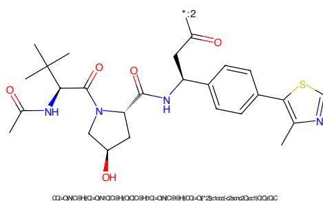
Figure 916: E3 - PROTAC ID: 687
