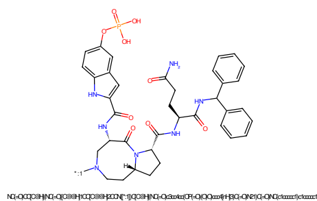
Figure 782: POI - PROTAC ID: 641
