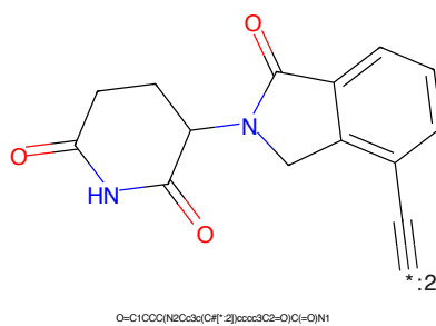
Figure 744: E3 - PROTAC ID: 630
