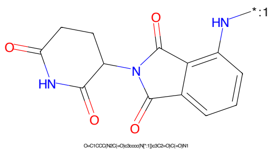
Figure 678: POI - PROTAC ID: 614
