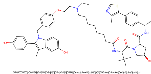
Figure 545: PROTAC - PROTAC ID: 540
