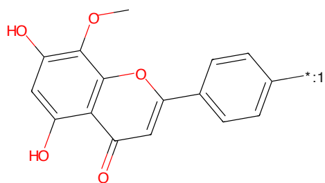
Figure 322: POI - PROTAC ID: 474
