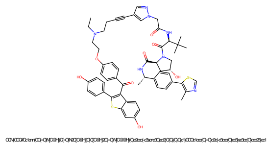
Figure 533: PROTAC - PROTAC ID: 536
