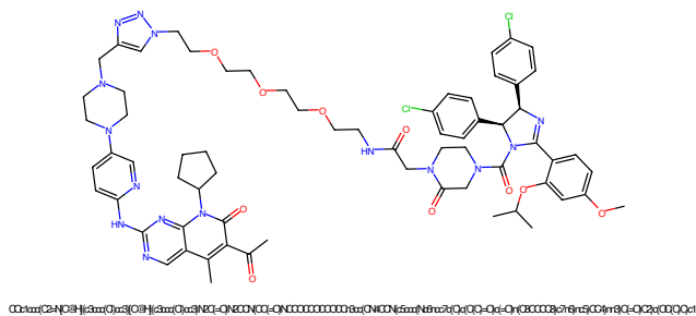
Figure 181: PROTAC - PROTAC ID: 431
