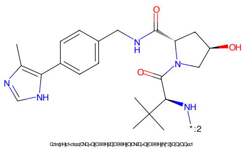
Figure 88: E3 - PROTAC ID: 399
