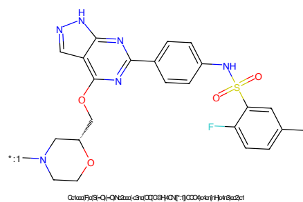
Figure 362: POI - PROTAC ID: 484
