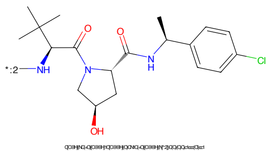
Figure 560: E3 - PROTAC ID: 543
