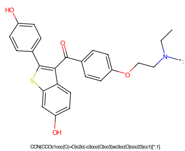
Figure 490: POI - PROTAC ID: 517
