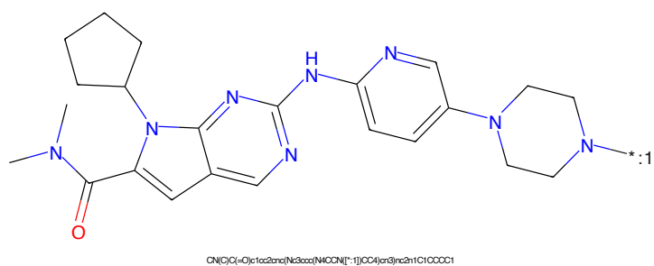
Figure 206: POI - PROTAC ID: 437
