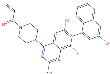
Figure 962: POI - PROTAC ID: 699
