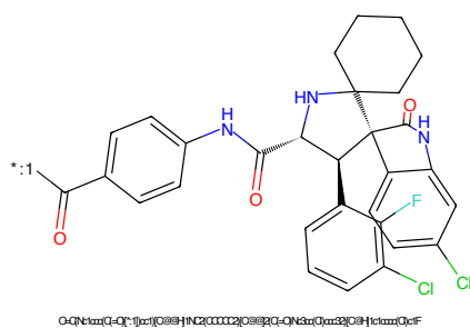
Figure 834: POI - PROTAC ID: 655
