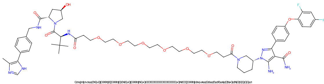
Figure 85: PROTAC - PROTAC ID: 399
