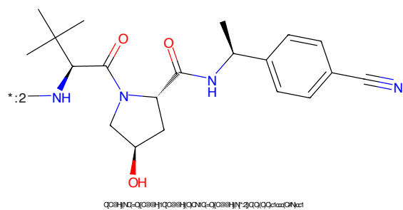
Figure 564: E3 - PROTAC ID: 544
