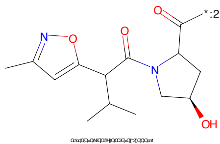
Figure 284: E3 - PROTAC ID: 462
