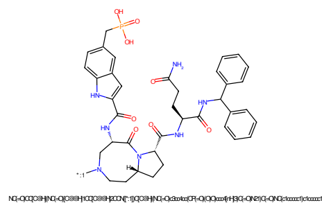
Figure 786: POI - PROTAC ID: 642
