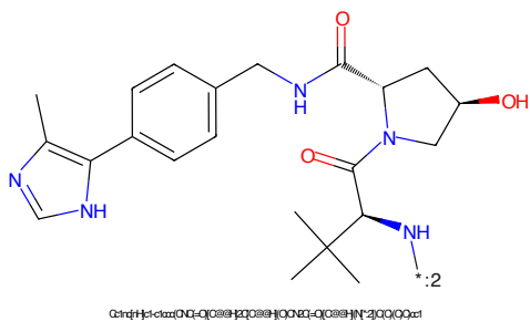
Figure 84: E3 - PROTAC ID: 398
