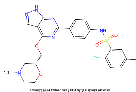
Figure 370: POI - PROTAC ID: 486
