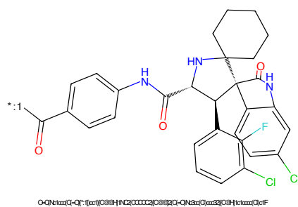
Figure 818: POI - PROTAC ID: 651
