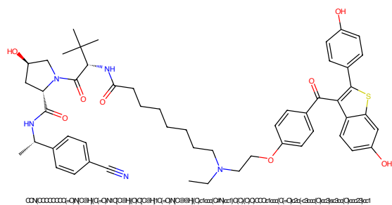
Figure 561: PROTAC - PROTAC ID: 544
