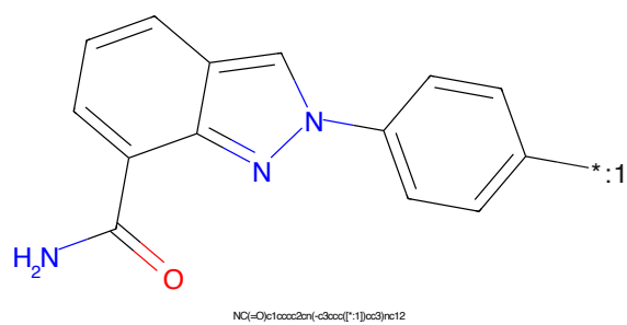
Figure 262: POI - PROTAC ID: 455
