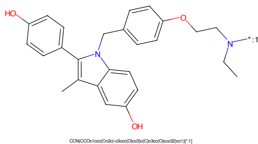
Figure 546: POI - PROTAC ID: 540
