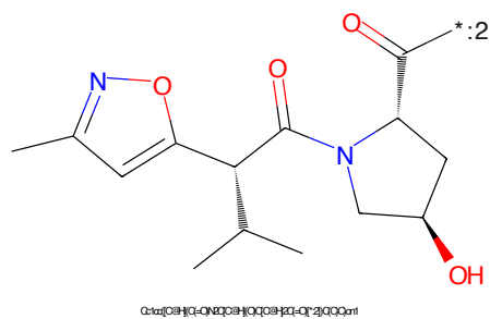
Figure 900: E3 - PROTAC ID: 683
