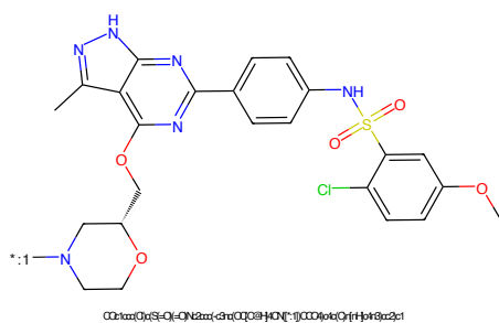
Figure 374: POI - PROTAC ID: 487
