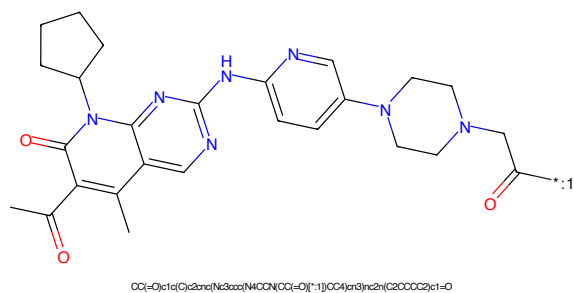
Figure 142: POI - PROTAC ID: 421
