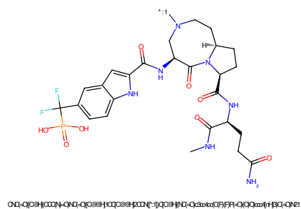
Figure 778: POI - PROTAC ID: 640
