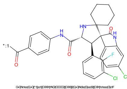
Figure 814: POI - PROTAC ID: 650
