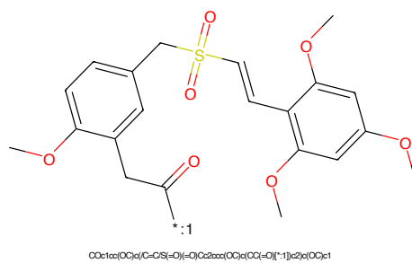
Figure 598: POI - PROTAC ID: 554
