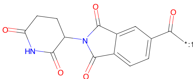
Figure 702: POI - PROTAC ID: 620
