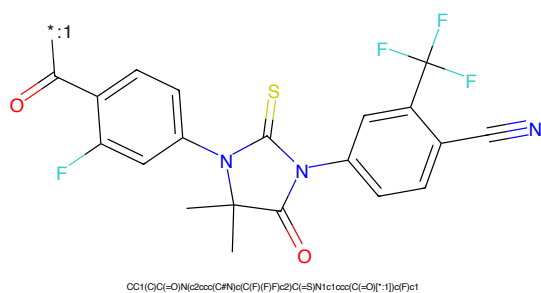
Figure 878: POI - PROTAC ID: 668
