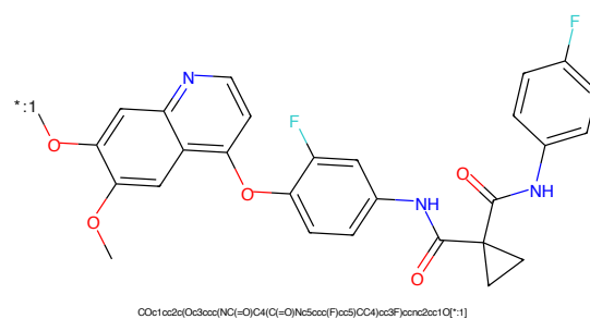
Figure 286: POI - PROTAC ID: 465
