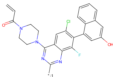
Figure 986: POI - PROTAC ID: 705
