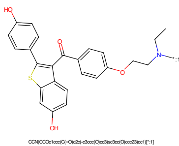
Figure 570: POI - PROTAC ID: 547
