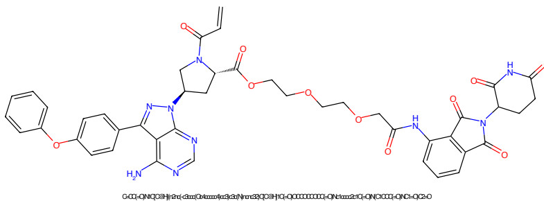
Figure 89: PROTAC - PROTAC ID: 400
