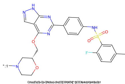
Figure 358: POI - PROTAC ID: 483
