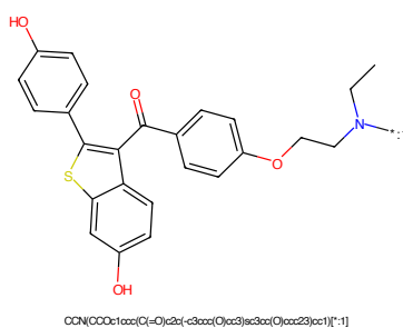
Figure 518: POI - PROTAC ID: 532
