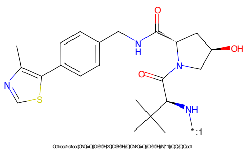
Figure 226: POI - PROTAC ID: 446
