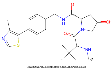
Figure 192: E3 - PROTAC ID: 433
