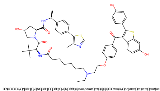
Figure 497: PROTAC - PROTAC ID: 519
