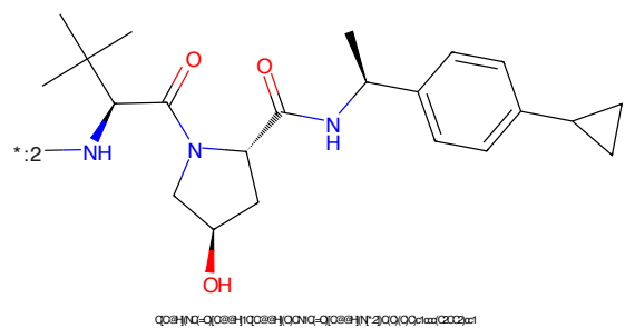
Figure 568: E3 - PROTAC ID: 546
