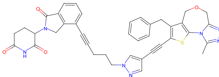
Figure 661: PROTAC - PROTAC ID: 577
