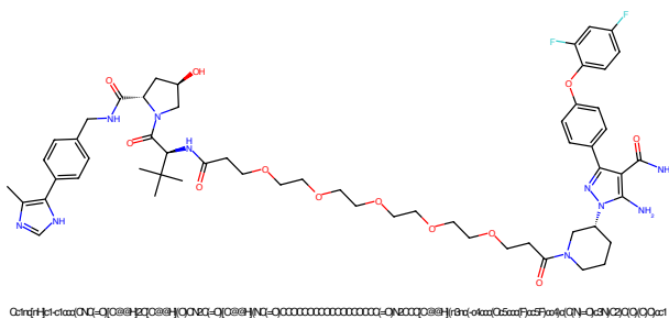
Figure 81: PROTAC - PROTAC ID: 398
