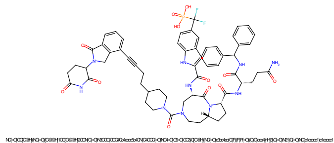
Figure 745: PROTAC - PROTAC ID: 631
