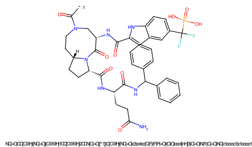
Figure 746: POI - PROTAC ID: 631
