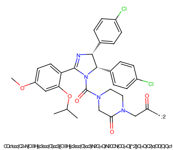
Figure 180: E3 - PROTAC ID: 430
