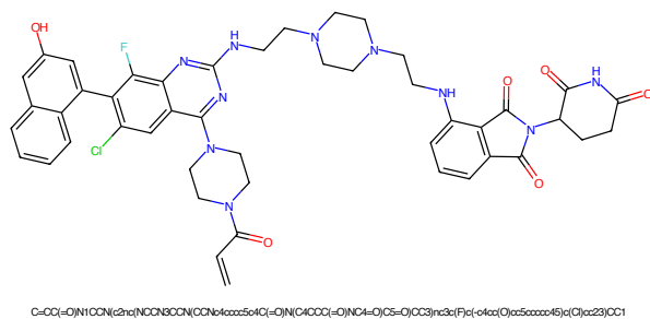
Figure 969: PROTAC - PROTAC ID: 701
