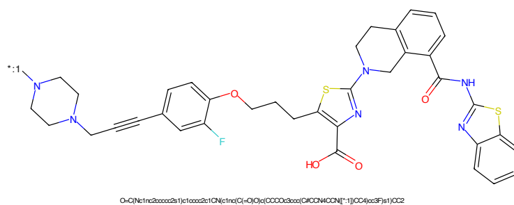
Figure 378: POI - PROTAC ID: 489
