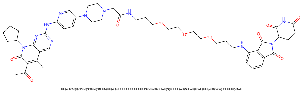
Figure 593: PROTAC - PROTAC ID: 553
