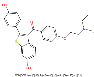
Figure 474: POI - PROTAC ID: 513
