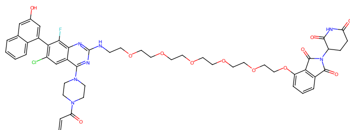
Figure 953: PROTAC - PROTAC ID: 697
