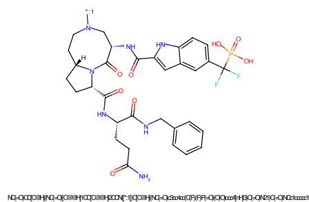
Figure 774: POI - PROTAC ID: 639
