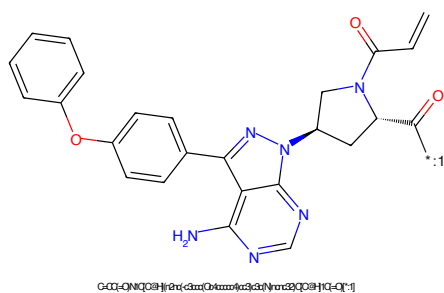
Figure 90: POI - PROTAC ID: 400
