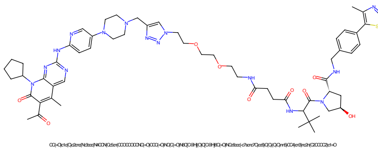
Figure 189: PROTAC - PROTAC ID: 433
