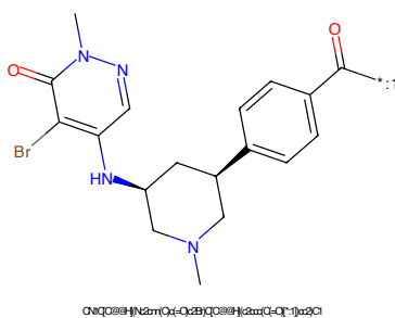
Figure 42: POI - PROTAC ID: 361
