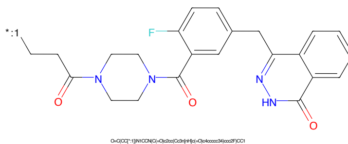
Figure 2: POI - PROTAC ID: 2089
