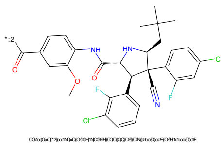
Figure 480: E3 - PROTAC ID: 3102
