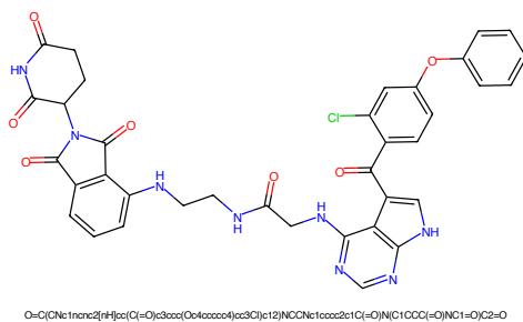
Figure 509: PROTAC - PROTAC ID: 3201
