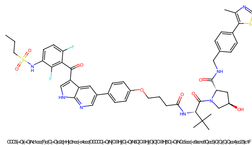
Figure 209: PROTAC - PROTAC ID: 2446
