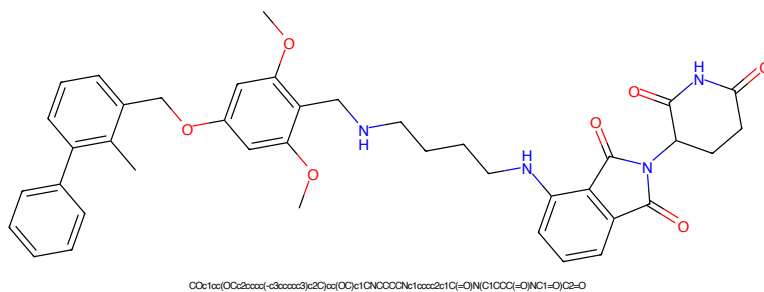
Figure 573: PROTAC - PROTAC ID: 3323
