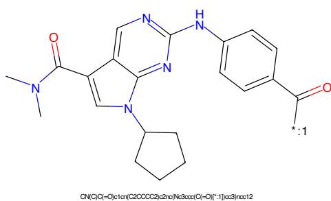
Figure 186: POI - PROTAC ID: 2333
