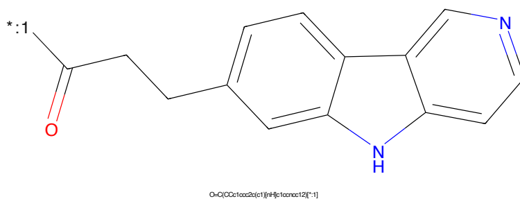
Figure 674: POI - PROTAC ID: 3572
