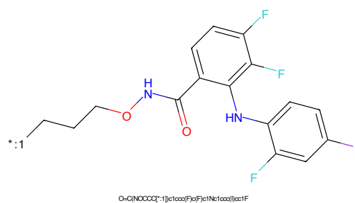
Figure 94: POI - PROTAC ID: 2143
