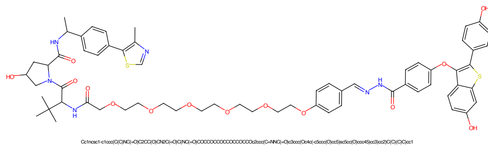
Figure 893: PROTAC - PROTAC ID: 1570
