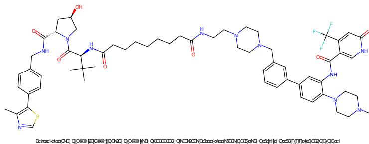
Figure 693: PROTAC - PROTAC ID: 3613
