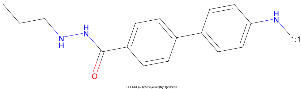
Figure 194: POI - PROTAC ID: 2388
