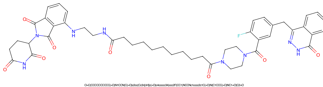
Figure 1: PROTAC - PROTAC ID: 2089
