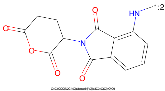
Figure 360: E3 - PROTAC ID: 2813
