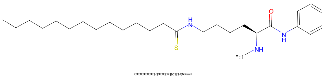
Figure 134: POI - PROTAC ID: 2221
