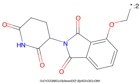
Figure 232: E3 - PROTAC ID: 2520
