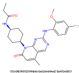
Figure 342: POI - PROTAC ID: 2734
