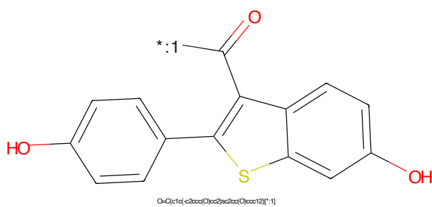
Figure 22: POI - PROTAC ID: 1616
