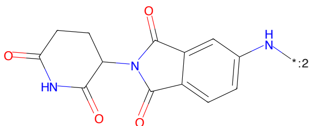
Figure 76: E3 - PROTAC ID: 1919
