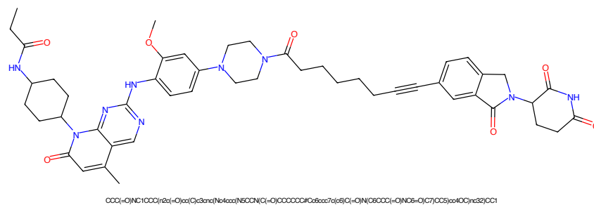
Figure 301: PROTAC - PROTAC ID: 2728
