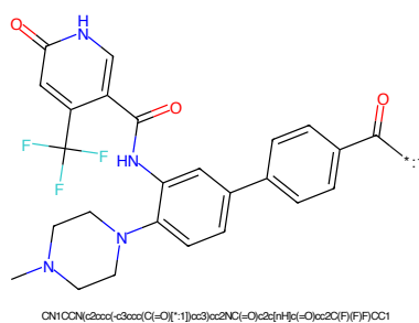
Figure 266: POI - PROTAC ID: 2659
