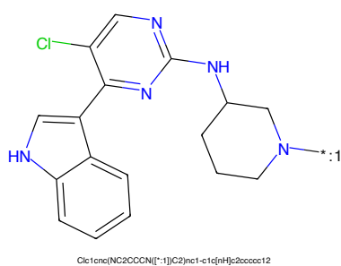
Figure 670: POI - PROTAC ID: 2622
