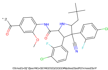
Figure 420: E3 - PROTAC ID: 3104
