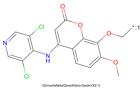
Figure 726: POI - PROTAC ID: 1681
