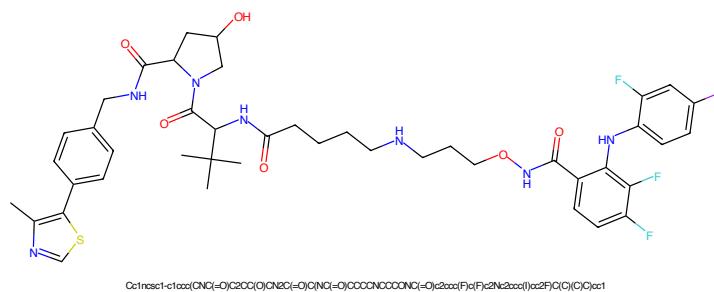
Figure 121: PROTAC - PROTAC ID: 2136
