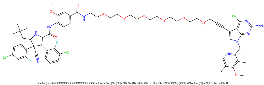
Figure 437: PROTAC - PROTAC ID: 3109
