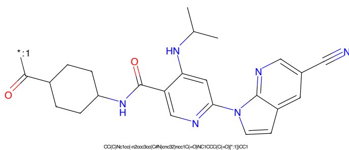
Figure 190: POI - PROTAC ID: 2378
