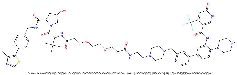
Figure 549: PROTAC - PROTAC ID: 3608
