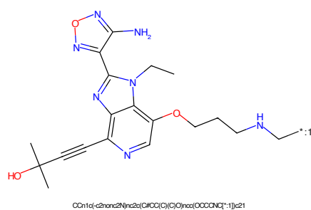
Figure 374: POI - PROTAC ID: 2954
