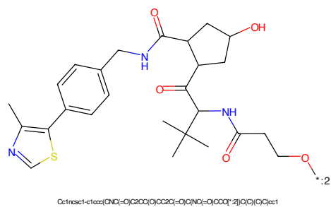
Figure 956: E3 - PROTAC ID: 3499
