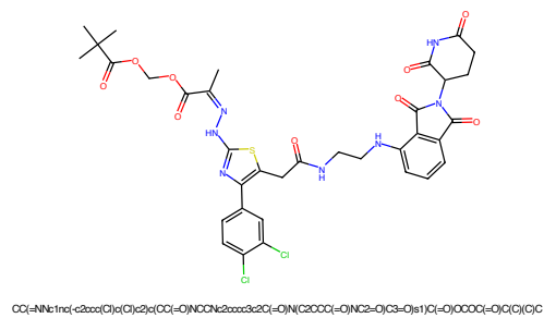
Figure 917: PROTAC - PROTAC ID: 3034
