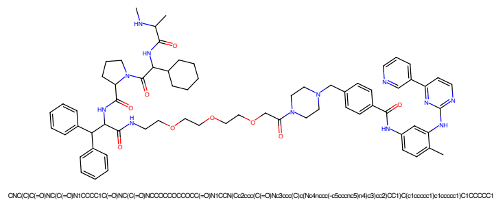
Figure 37: PROTAC - PROTAC ID: 1661
