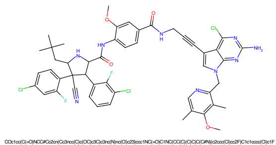
Figure 401: PROTAC - PROTAC ID: 3100
