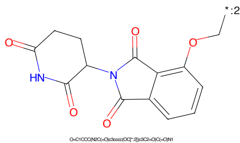
Figure 388: E3 - PROTAC ID: 3063
