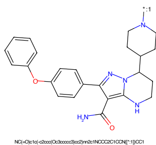
Figure 494: POI - PROTAC ID: 3456
