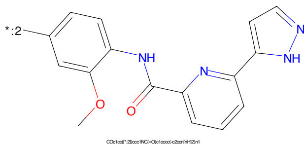
Figure 992: E3 - PROTAC ID: 3441
