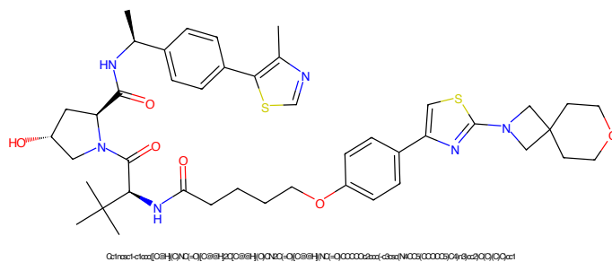
Figure 805: PROTAC - PROTAC ID: 3402
