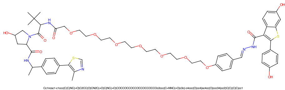
Figure 33: PROTAC - PROTAC ID: 1619
