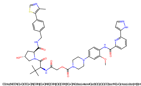
Figure 813: PROTAC - PROTAC ID: 3437
