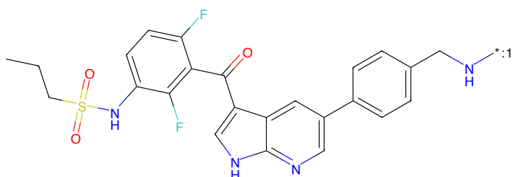
Figure 50: POI - PROTAC ID: 1741
