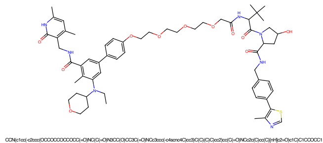
Figure 341: PROTAC - PROTAC ID: 2823
