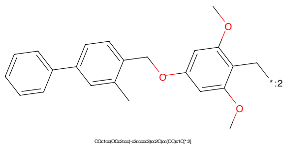
Figure 792: E3 - PROTAC ID: 3332
