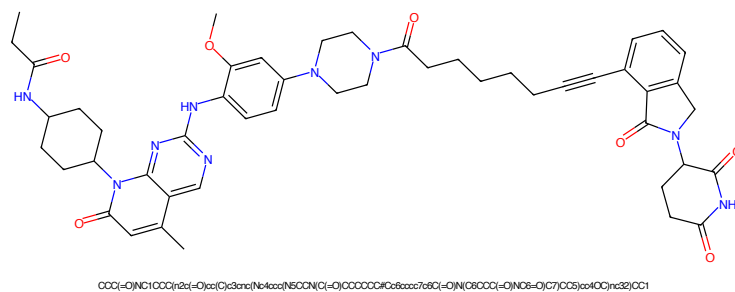
Figure 313: PROTAC - PROTAC ID: 2732
