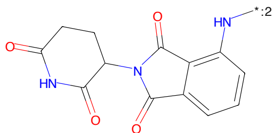
Figure 72: E3 - PROTAC ID: 1914
