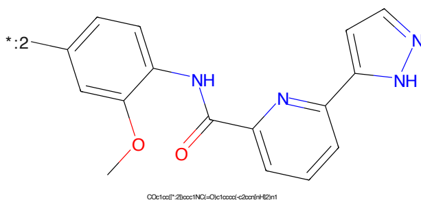
Figure 988: E3 - PROTAC ID: 3440
