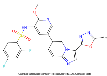
Figure 474: POI - PROTAC ID: 3295
