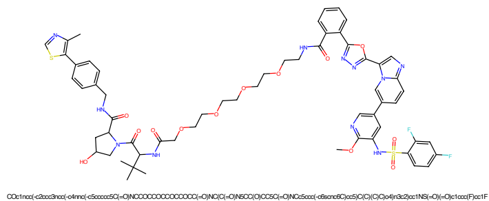
Figure 473: PROTAC - PROTAC ID: 3295
