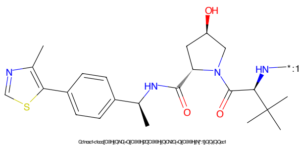
Figure 806: POI - PROTAC ID: 3402
