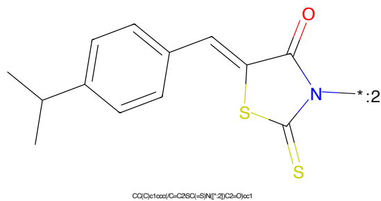
Figure 784: E3 - PROTAC ID: 3316
