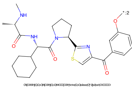
Figure 728: E3 - PROTAC ID: 1681
