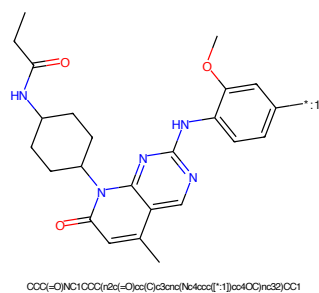
Figure 306: POI - PROTAC ID: 2729
