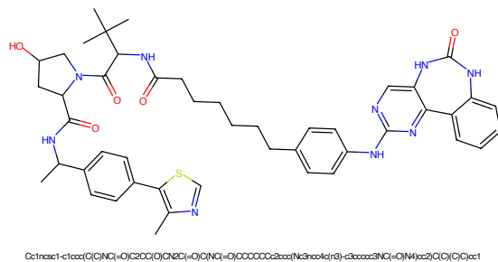
Figure 913: PROTAC - PROTAC ID: 2548
