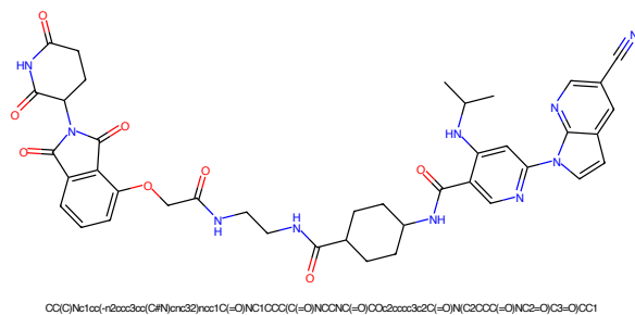
Figure 181: PROTAC - PROTAC ID: 2376
