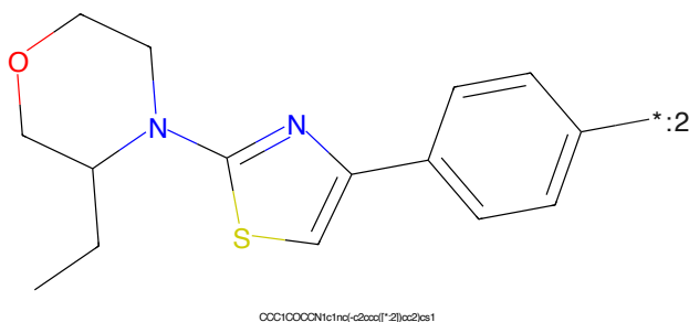
Figure 796: E3 - PROTAC ID: 3398
