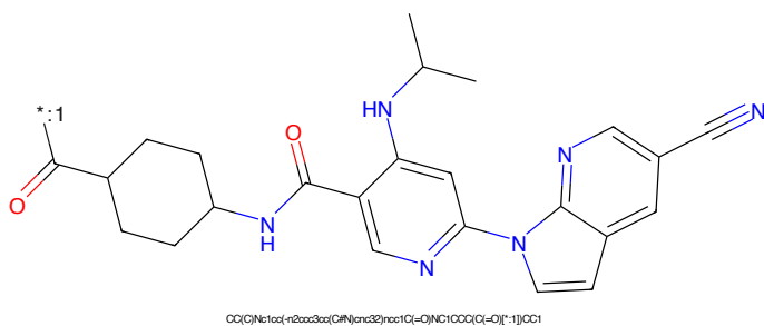
Figure 194: POI - PROTAC ID: 2379
