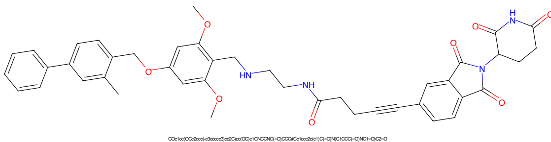
Figure 785: PROTAC - PROTAC ID: 3329
