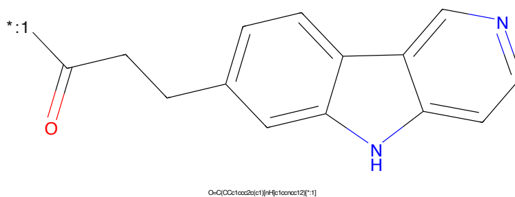
Figure 546: POI - PROTAC ID: 3575
