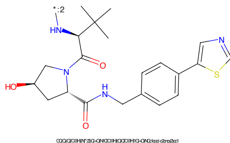
Figure 748: E3 - PROTAC ID: 1948
