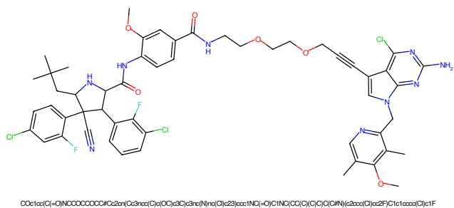
Figure 421: PROTAC - PROTAC ID: 3105
