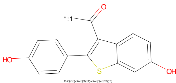
Figure 10: POI - PROTAC ID: 1611
