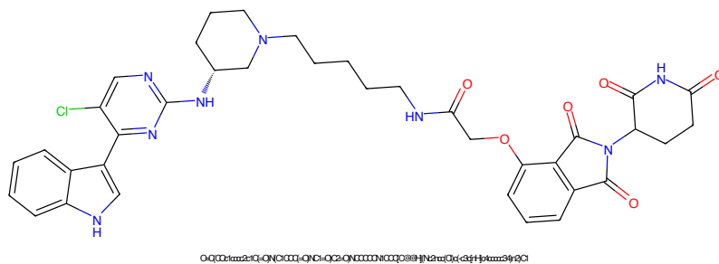
Figure 633: PROTAC - PROTAC ID: 2620
