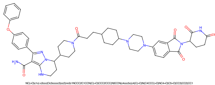
Figure 513: PROTAC - PROTAC ID: 3462
