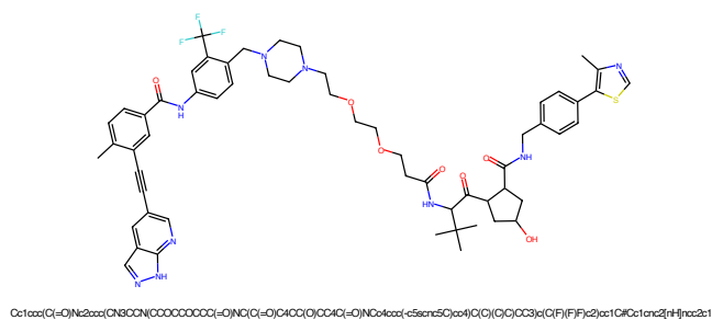
Figure 953: PROTAC - PROTAC ID: 3499
