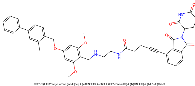
Figure 789: PROTAC - PROTAC ID: 3332
