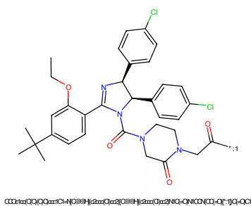
Figure 862: POI - PROTAC ID: 3493
