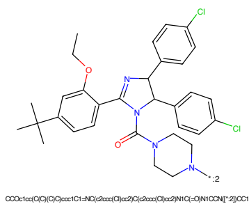
Figure 832: E3 - PROTAC ID: 3485
