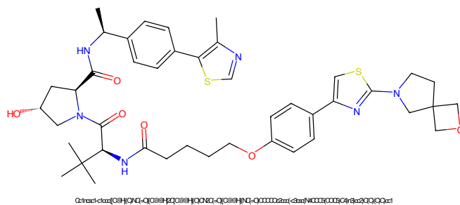
Figure 801: PROTAC - PROTAC ID: 3401
