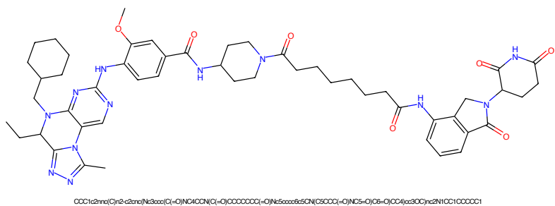
Figure 397: PROTAC - PROTAC ID: 3069
