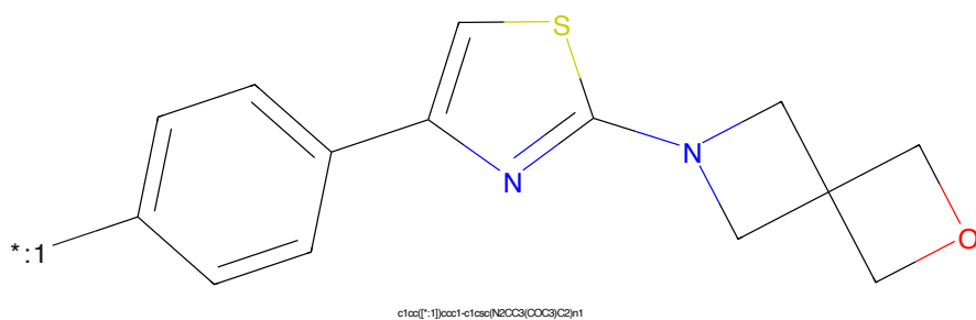
Figure 930: POI - PROTAC ID: 3400
