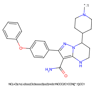
Figure 506: POI - PROTAC ID: 3460
