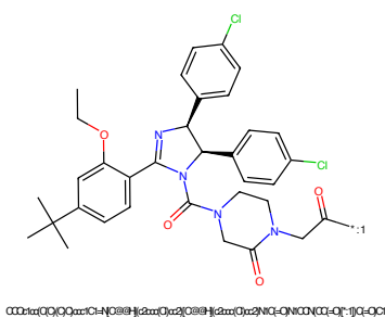
Figure 870: POI - PROTAC ID: 3495
