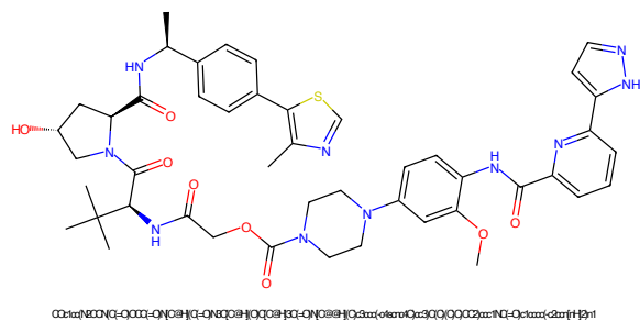
Figure 817: PROTAC - PROTAC ID: 3438
