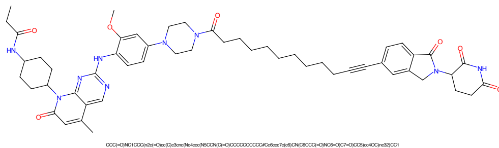
Figure 297: PROTAC - PROTAC ID: 2726
