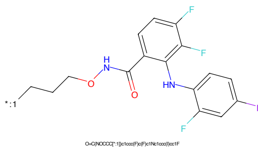
Figure 158: POI - PROTAC ID: 2149
