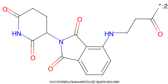
Figure 772: E3 - PROTAC ID: 2467
