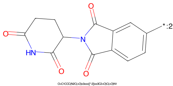
Figure 600: E3 - PROTAC ID: 2902
