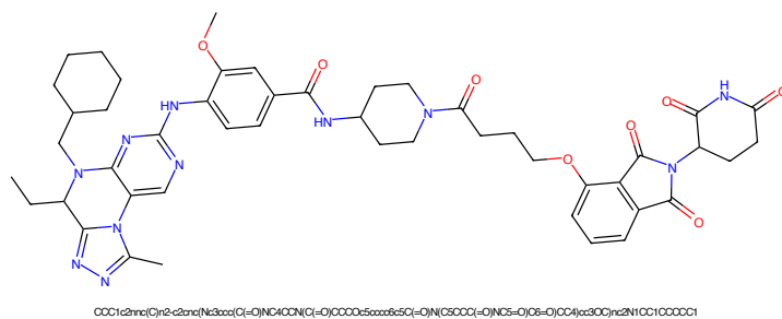
Figure 381: PROTAC - PROTAC ID: 3062
