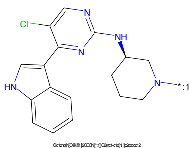
Figure 630: POI - PROTAC ID: 2619
