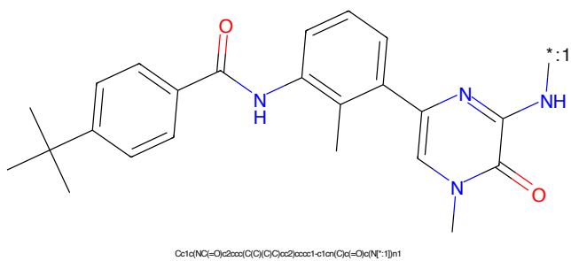
Figure 738: POI - PROTAC ID: 1795
