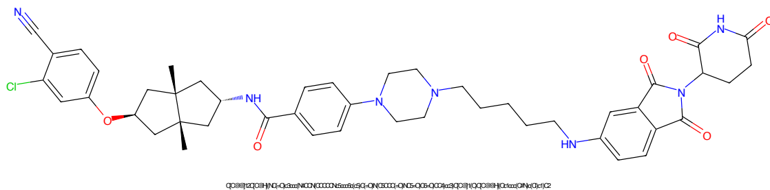
Figure 937: PROTAC - PROTAC ID: 2279
