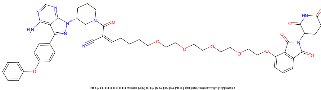
Figure 281: PROTAC - PROTAC ID: 1902
