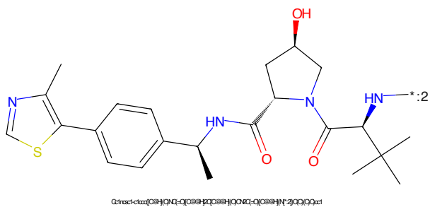
Figure 476: E3 - PROTAC ID: 1999
