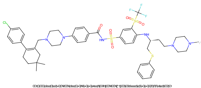
Figure 238: POI - PROTAC ID: 1880
