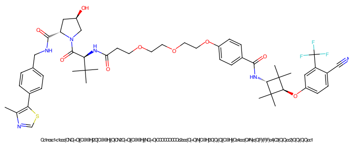
Figure 613: PROTAC - PROTAC ID: 2043
