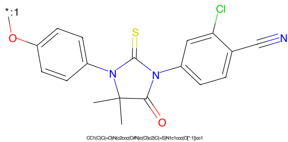
Figure 650: POI - PROTAC ID: 2064
