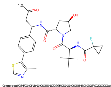
Figure 952: E3 - PROTAC ID: 2282
