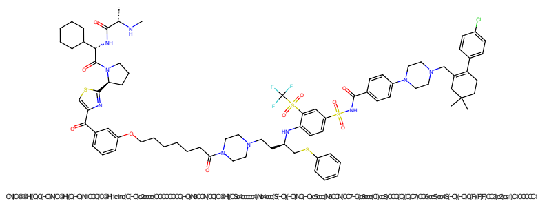
Figure 33: PROTAC - PROTAC ID: 1808
