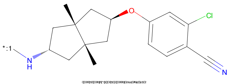
Figure 942: POI - PROTAC ID: 2280
