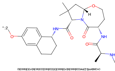
Figure 56: E3 - PROTAC ID: 1813
