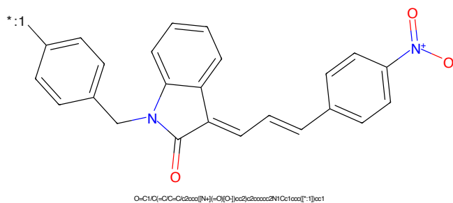
Figure 634: POI - PROTAC ID: 2048
