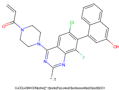
Figure 470: POI - PROTAC ID: 1997
