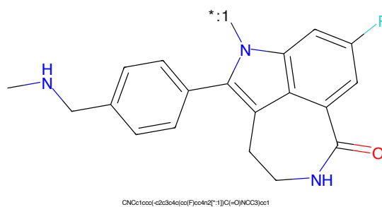
Figure 98: POI - PROTAC ID: 1824
