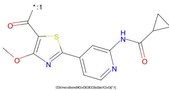
Figure 998: POI - PROTAC ID: 2294
