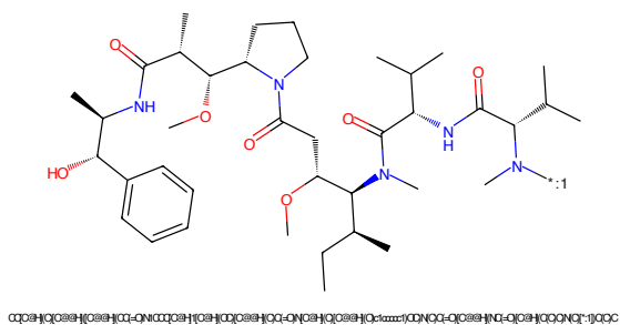
Figure 174: POI - PROTAC ID: 1862
