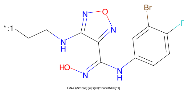
Figure 782: POI - PROTAC ID: 2225
