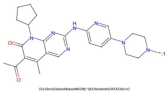
Figure 334: POI - PROTAC ID: 1940
