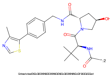
Figure 304: E3 - PROTAC ID: 1907
