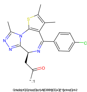
Figure 658: POI - PROTAC ID: 2067
