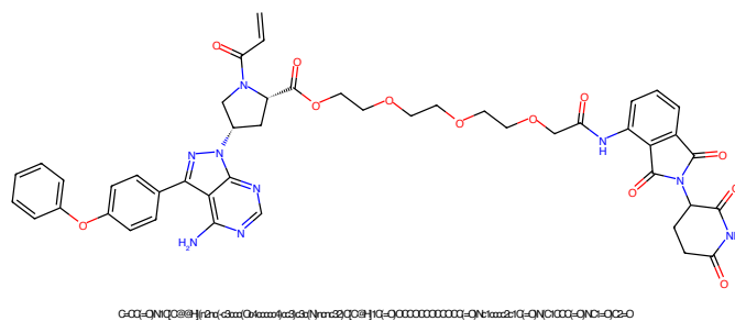
Figure 245: PROTAC - PROTAC ID: 1882
