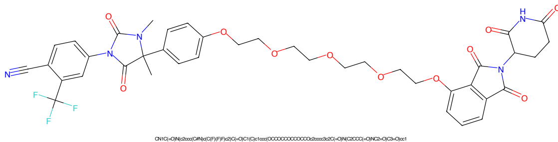
Figure 589: PROTAC - PROTAC ID: 2033
