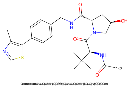
Figure 308: E3 - PROTAC ID: 1908
