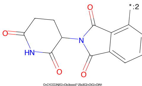
Figure 872: E3 - PROTAC ID: 2262
