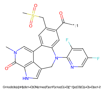
Figure 758: POI - PROTAC ID: 2202
