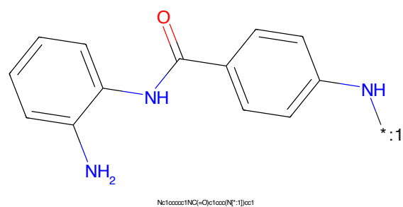
Figure 854: POI - PROTAC ID: 2258
