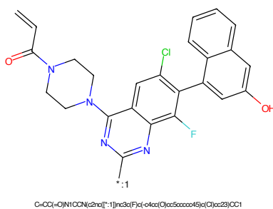
Figure 462: POI - PROTAC ID: 1995
