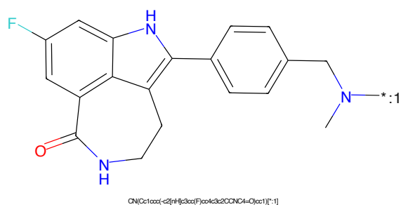
Figure 110: POI - PROTAC ID: 1827
