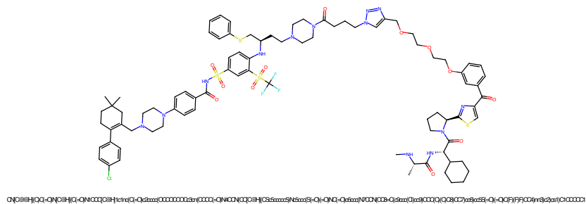
Figure 5: PROTAC - PROTAC ID: 1801
