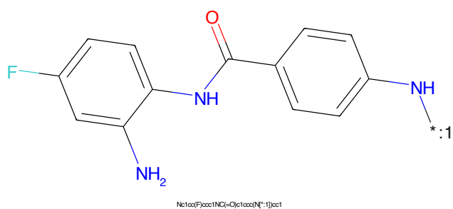
Figure 866: POI - PROTAC ID: 2261
