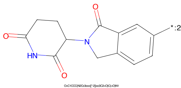
Figure 440: E3 - PROTAC ID: 1982
