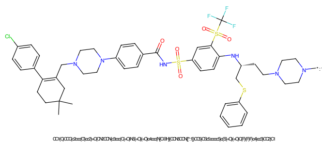
Figure 10: POI - PROTAC ID: 1802
