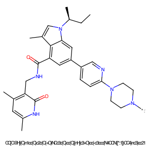
Figure 742: POI - PROTAC ID: 2181
