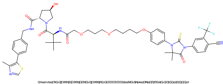
Figure 597: PROTAC - PROTAC ID: 2037
