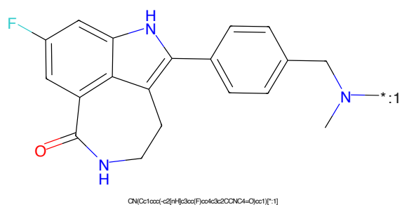
Figure 70: POI - PROTAC ID: 1817
