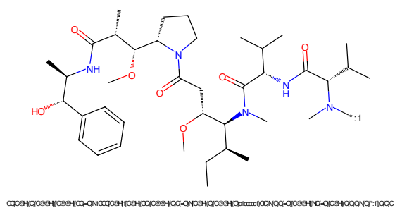
Figure 190: POI - PROTAC ID: 1866
