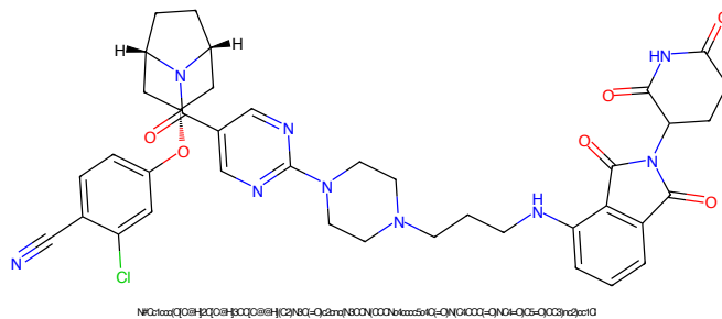
Figure 889: PROTAC - PROTAC ID: 2267
