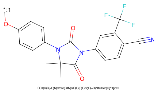
Figure 358: POI - PROTAC ID: 1946
