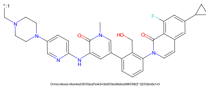
Figure 2: POI - PROTAC ID: 1799
