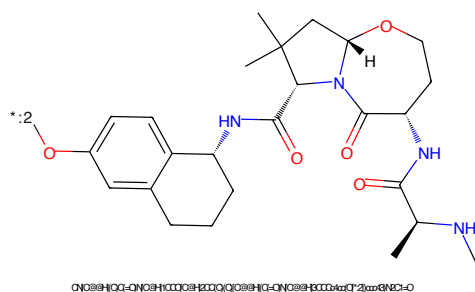
Figure 60: E3 - PROTAC ID: 1814
