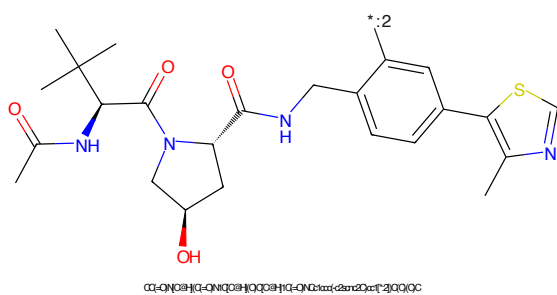
Figure 220: E3 - PROTAC ID: 2809
