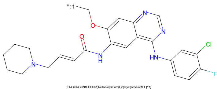
Figure 78: POI - PROTAC ID: 2774
