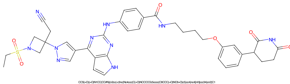
Figure 977: PROTAC - PROTAC ID: 3225
