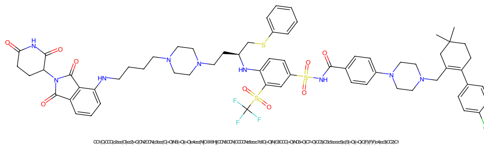
Figure 121: PROTAC - PROTAC ID: 31
