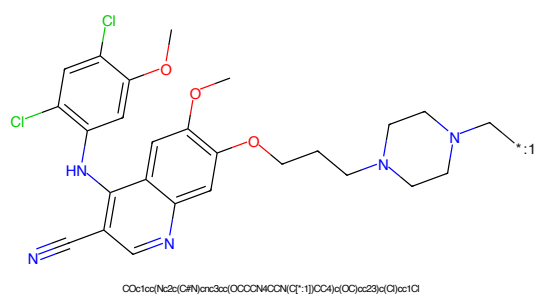
Figure 418: POI - PROTAC ID: 158
