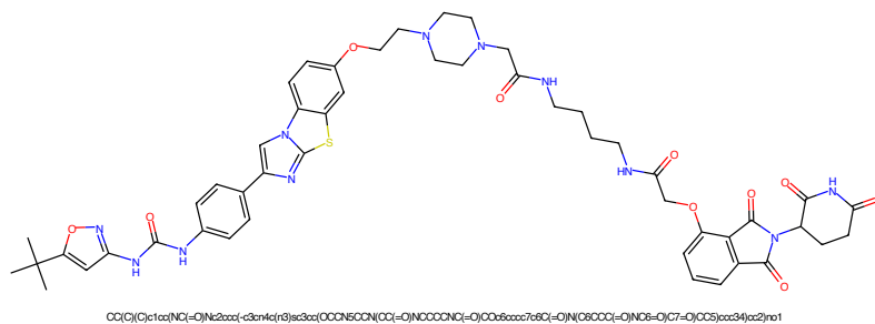
Figure 401: PROTAC - PROTAC ID: 154
