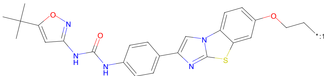
Figure 394: POI - PROTAC ID: 152
