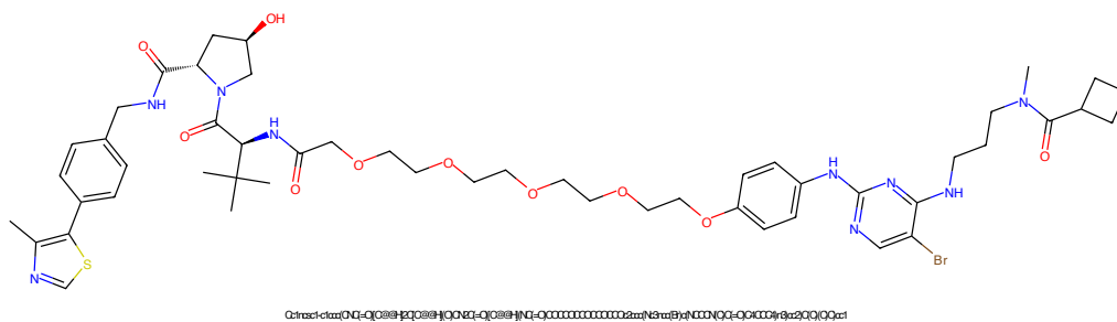
Figure 449: PROTAC - PROTAC ID: 167
