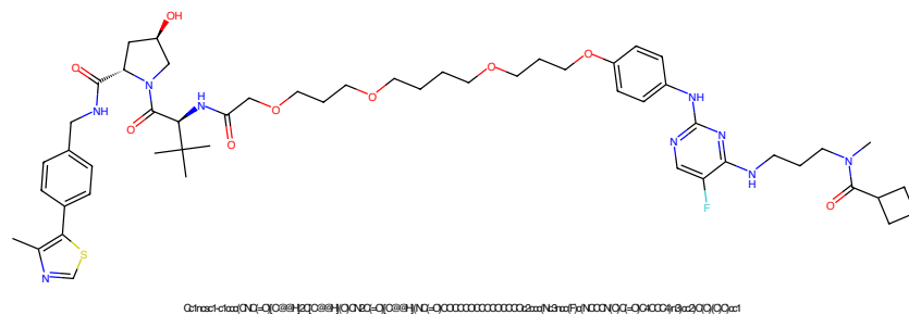
Figure 489: PROTAC - PROTAC ID: 177
