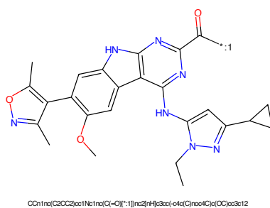
Figure 310: POI - PROTAC ID: 108
