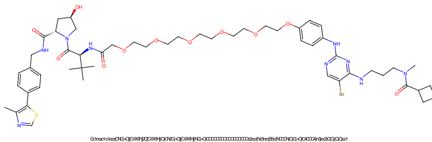
Figure 461: PROTAC - PROTAC ID: 170
