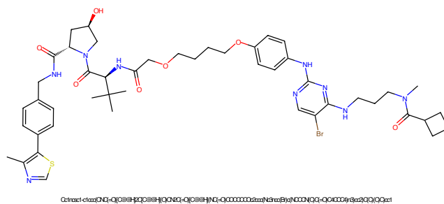
Figure 421: PROTAC - PROTAC ID: 160
