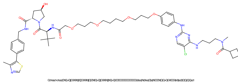
Figure 493: PROTAC - PROTAC ID: 178
