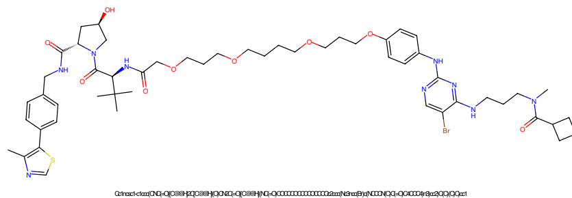
Figure 453: PROTAC - PROTAC ID: 168
