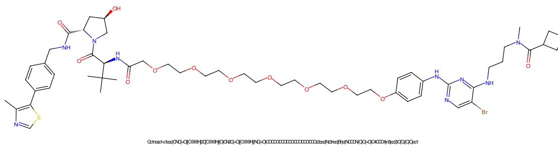
Figure 473: PROTAC - PROTAC ID: 173
