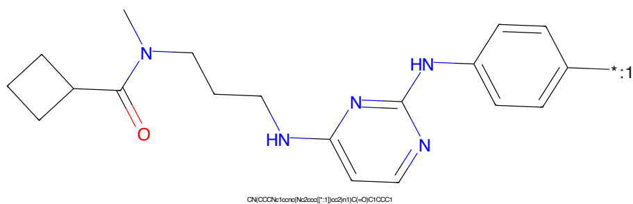
Figure 486: POI - PROTAC ID: 176
