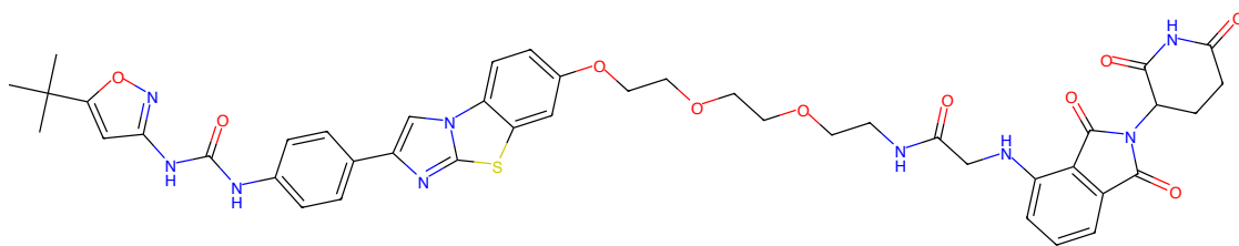
Figure 393: PROTAC - PROTAC ID: 152
