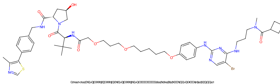
Figure 441: PROTAC - PROTAC ID: 165
