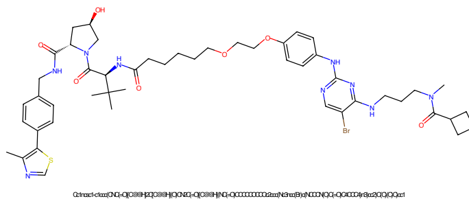
Figure 429: PROTAC - PROTAC ID: 162
