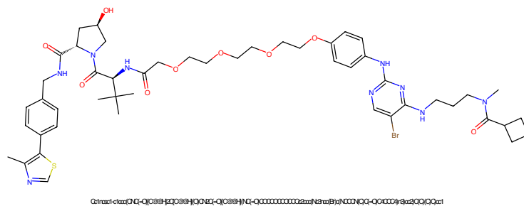
Figure 437: PROTAC - PROTAC ID: 164
