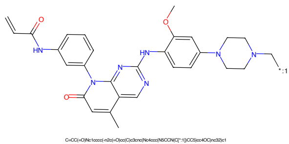
Figure 234: POI - PROTAC ID: 69
