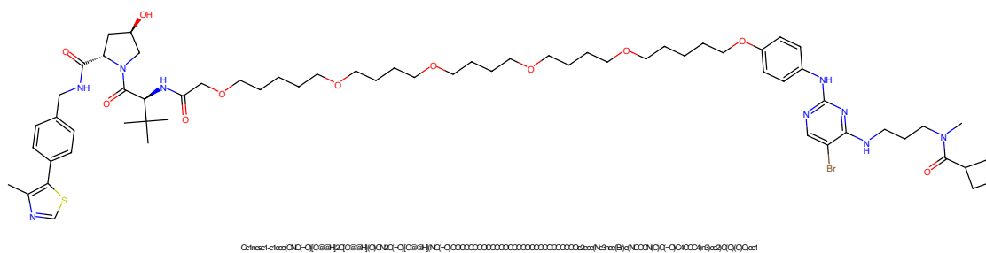
Figure 481: PROTAC - PROTAC ID: 175
