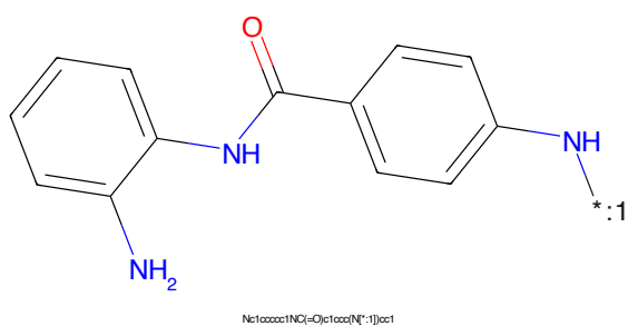
Figure 378: POI - PROTAC ID: 2257
