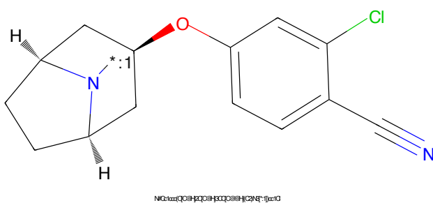
Figure 414: POI - PROTAC ID: 2266
