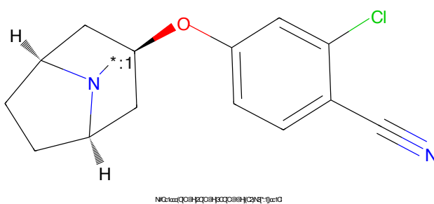
Figure 402: POI - PROTAC ID: 2263
