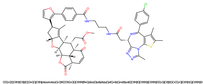
Figure 197: PROTAC - PROTAC ID: 2067
