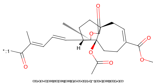
Figure 358: POI - PROTAC ID: 2245
