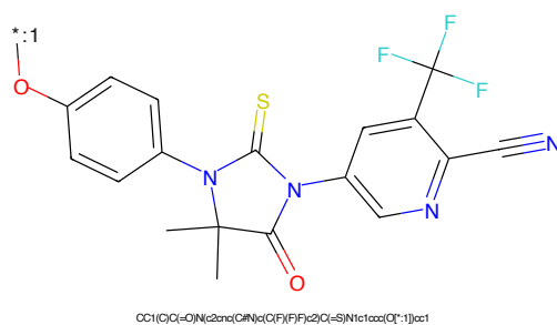
Figure 178: POI - PROTAC ID: 2059
