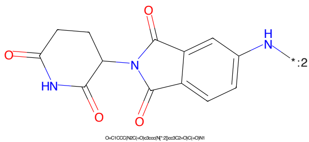
Figure 460: E3 - PROTAC ID: 2277
