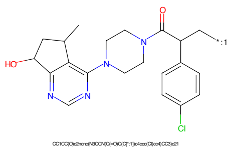
Figure 2: POI - PROTAC ID: 2941
