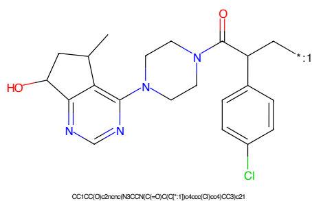
Figure 6: POI - PROTAC ID: 2942
