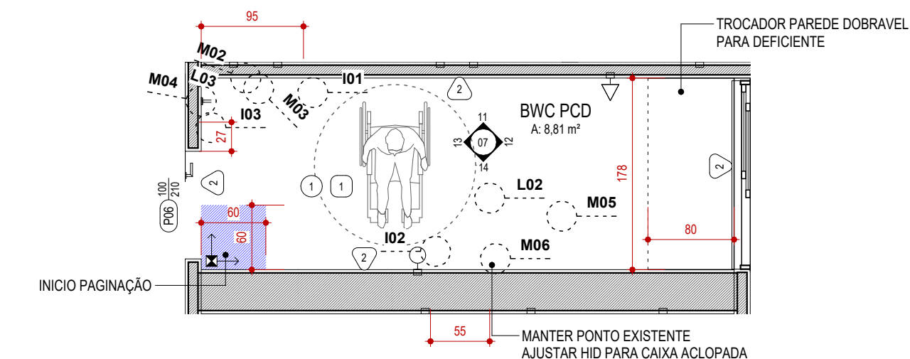
10 PLANTA BANHEIRO PCD 1 : 50
