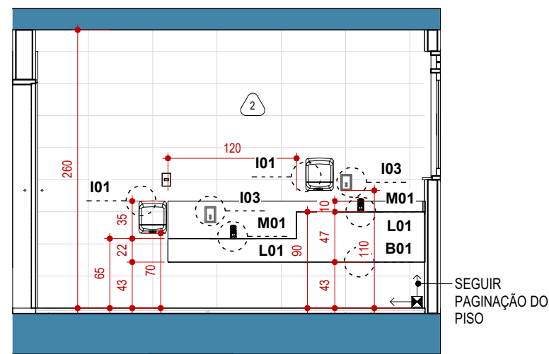
4 ELEV FEM 1 : 50
