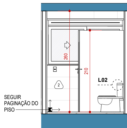
7 ELEV MASC 1 : 50
