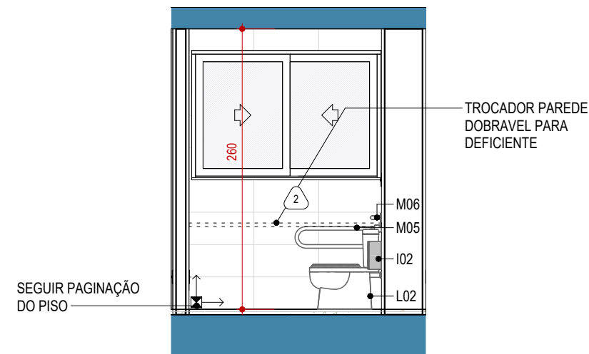
12 ELEV PCD 1 : 50
