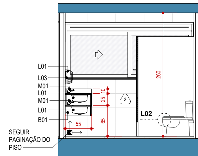
5 ELEV FEM 1 : 50
