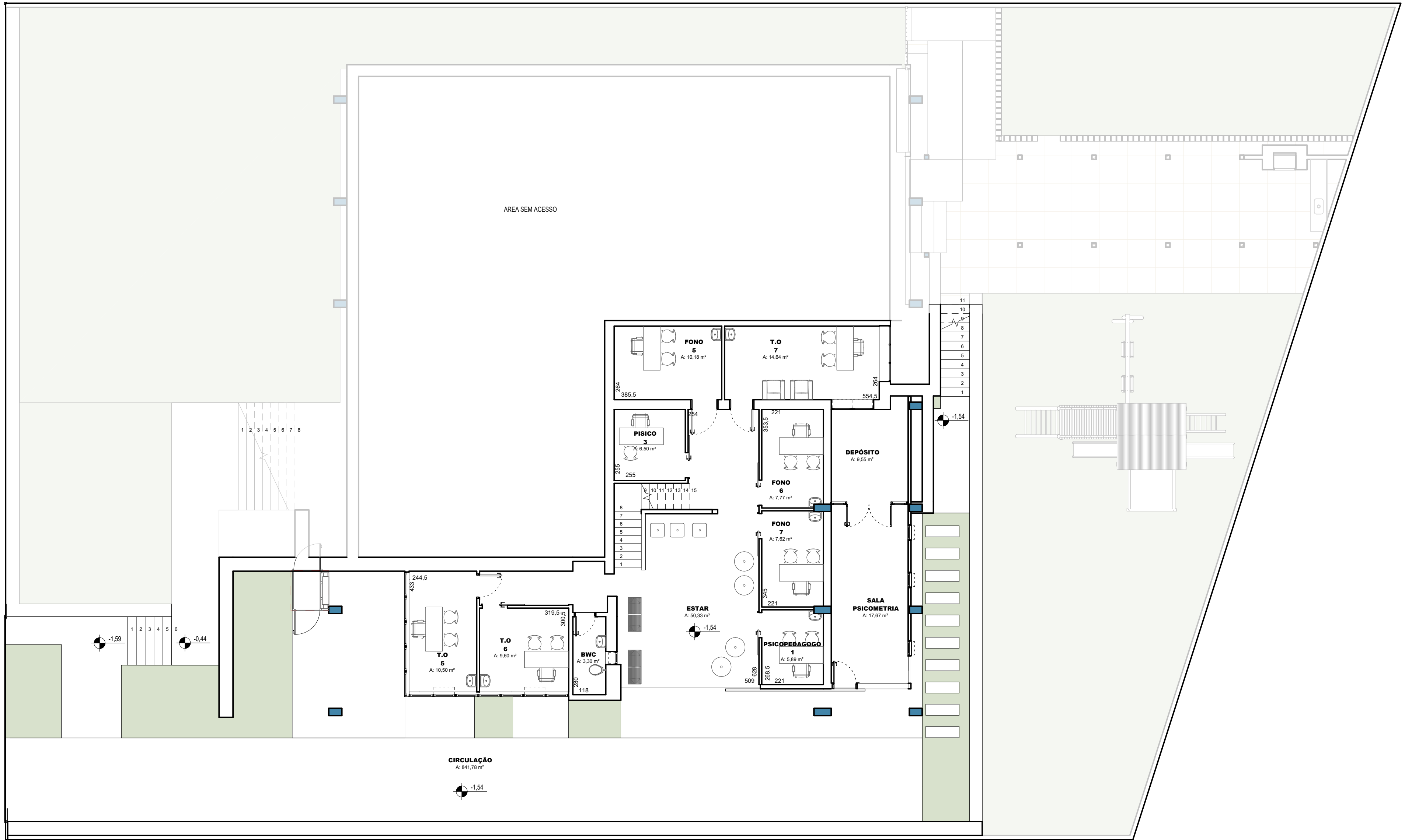
1 PLANTA INFERIOR - LAYOUT 1 : 100
