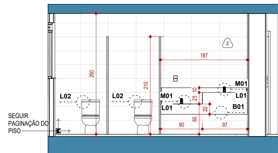
8 ELEV MASC 1 : 50
