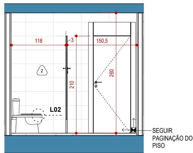
3 ELEV FEM 1 : 50
