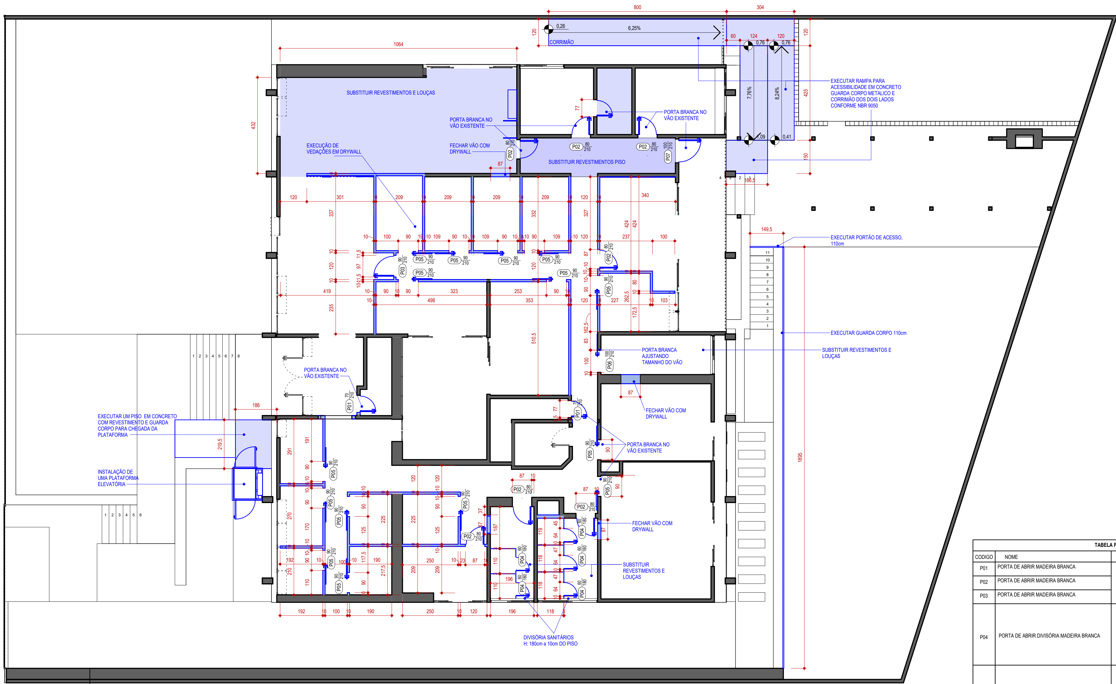
1 PLANTA A CONSTRUIR 1 : 100
