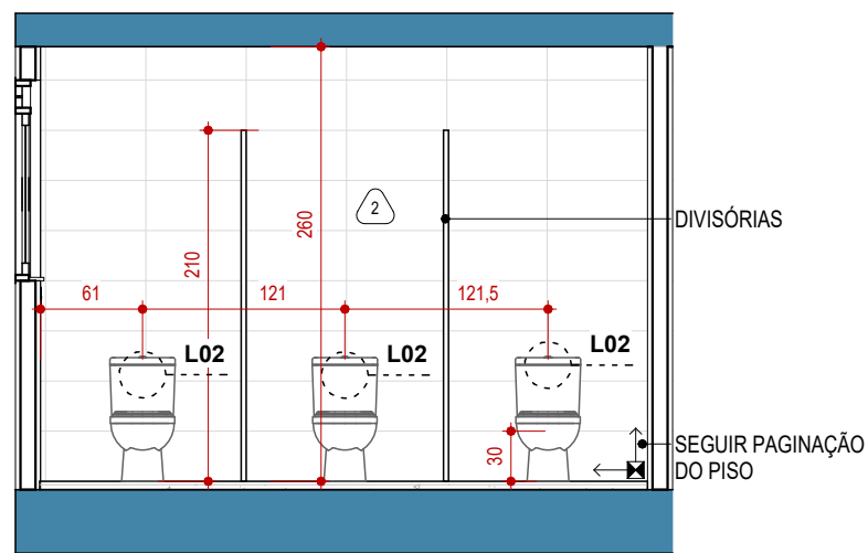
2 ELEV FEM 1 : 50
