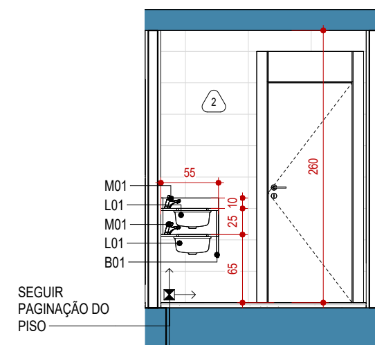
9 ELEV MASC 1 : 50
