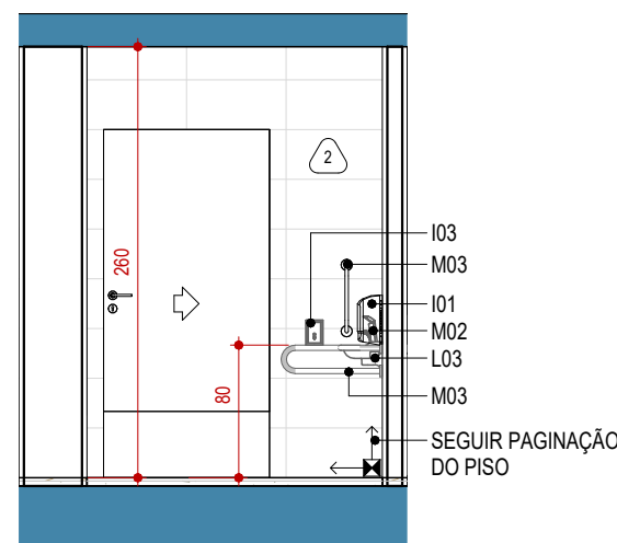
13 ELEV PCD 1 : 50
