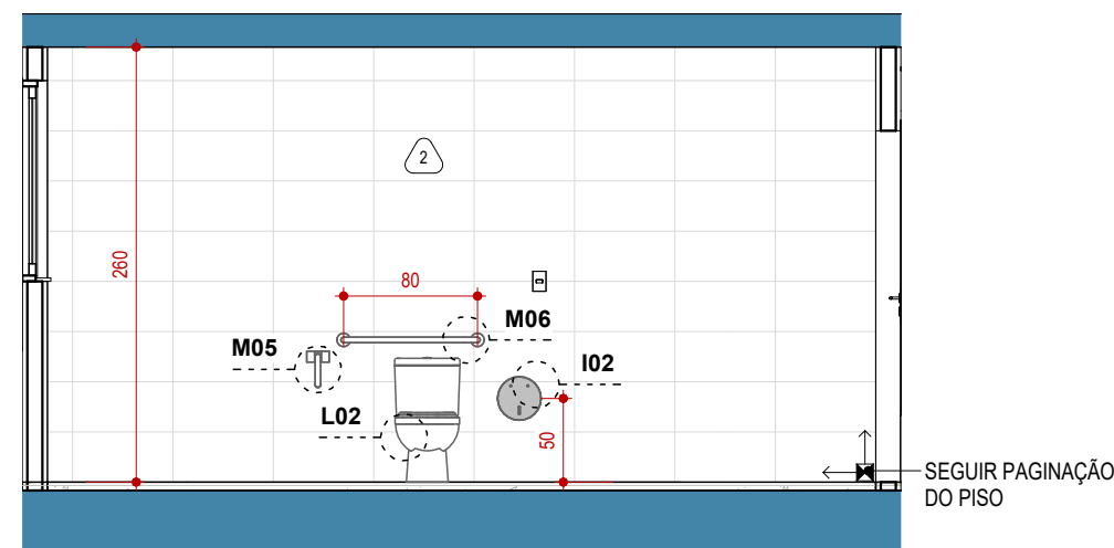
14 ELEV PCD 1 : 50
