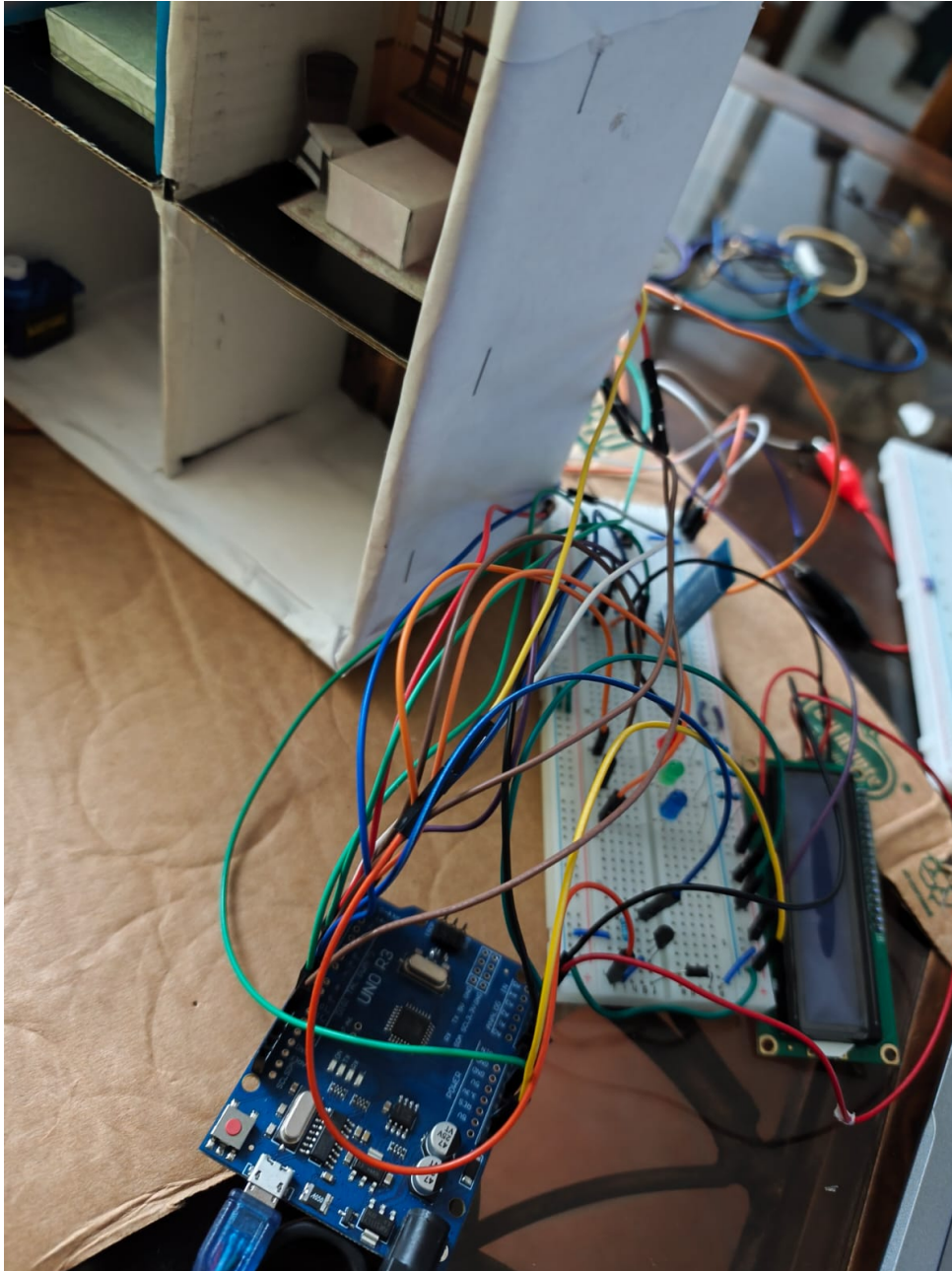
Figure 28: Vista lateral del cableado entre la maqueta, el Arduino y el módulo LCD.
