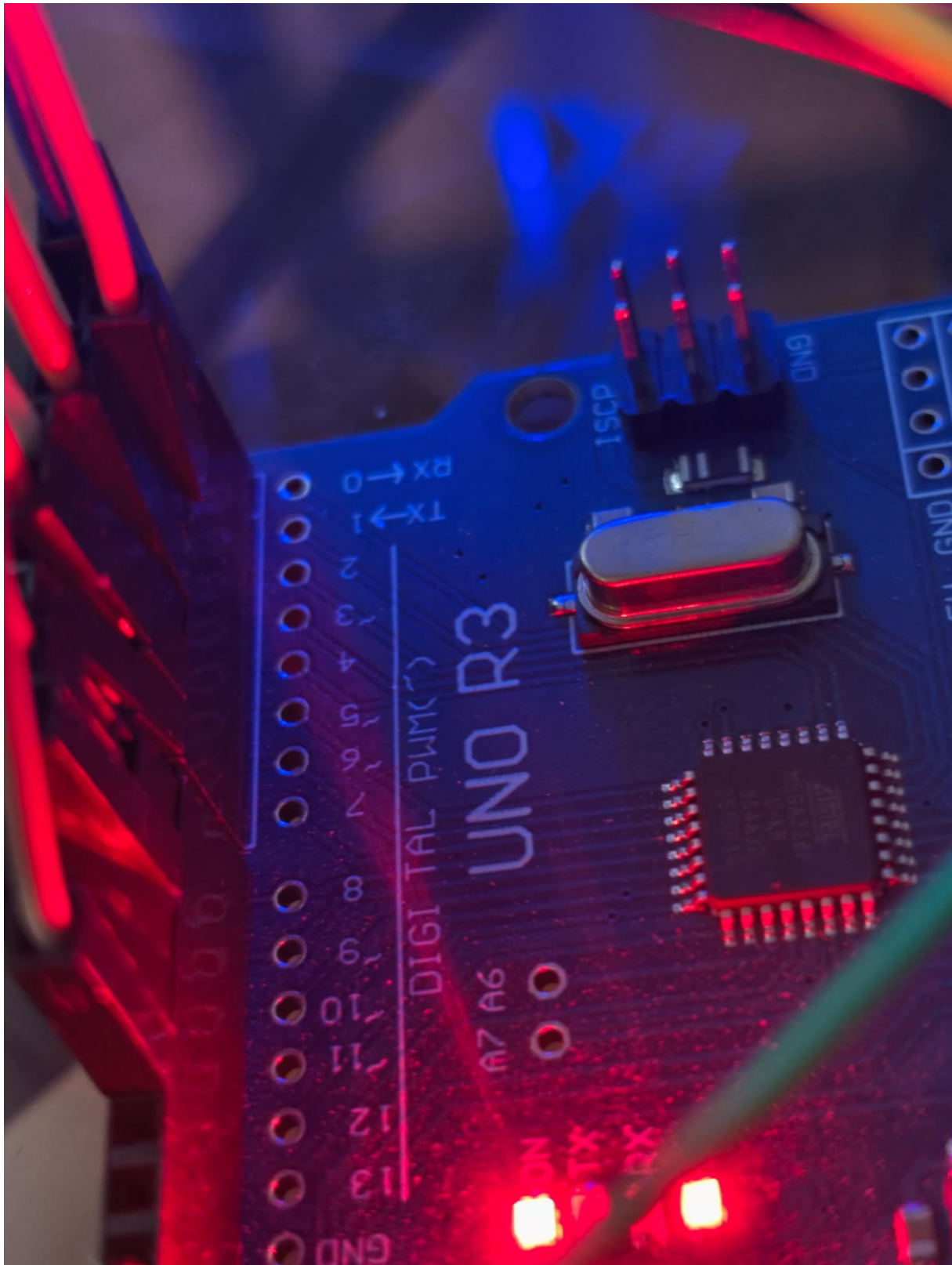
Figure 26: Maqueta física en funcionamiento con iluminación activa y mecanismo de puerta en prueba.
