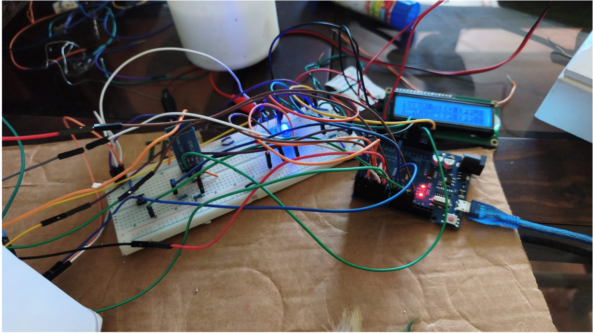
Figure 27: Montaje general con Arduino, protoboard de control y LCD I2C conectados.
