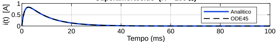
Superamortecido ( R = 100 \Omega )
