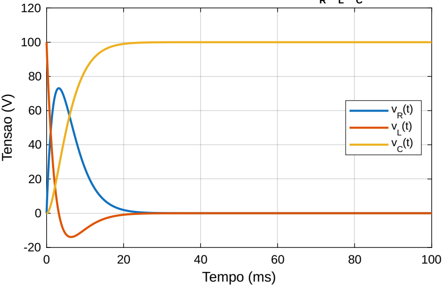
Criticamente Amortecido ( R = 62\ \Omega ) - v_R , v_L , v_C
