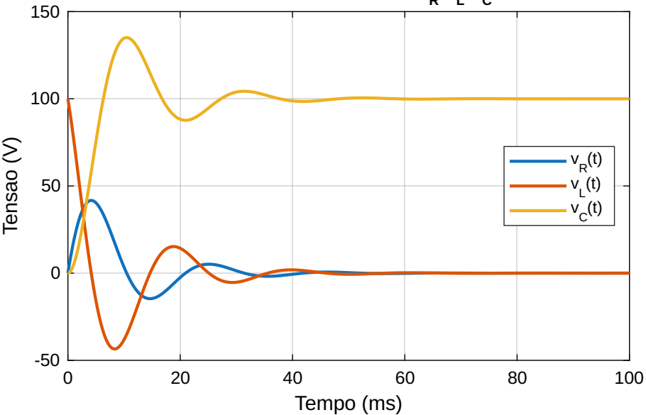
Subamortecido ( R = 20\ \Omega ) - v_R , v_L , v_C
