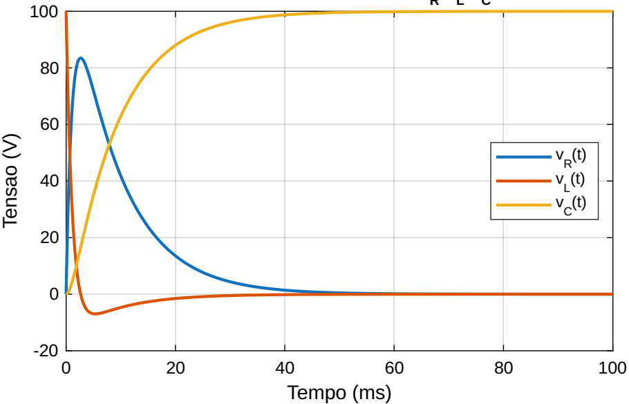
Superamortecido ( R = 100\ \Omega ) - v_R , v_L , v_C
